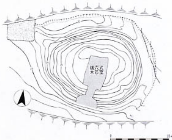
墳丘測量図 (1:400)
