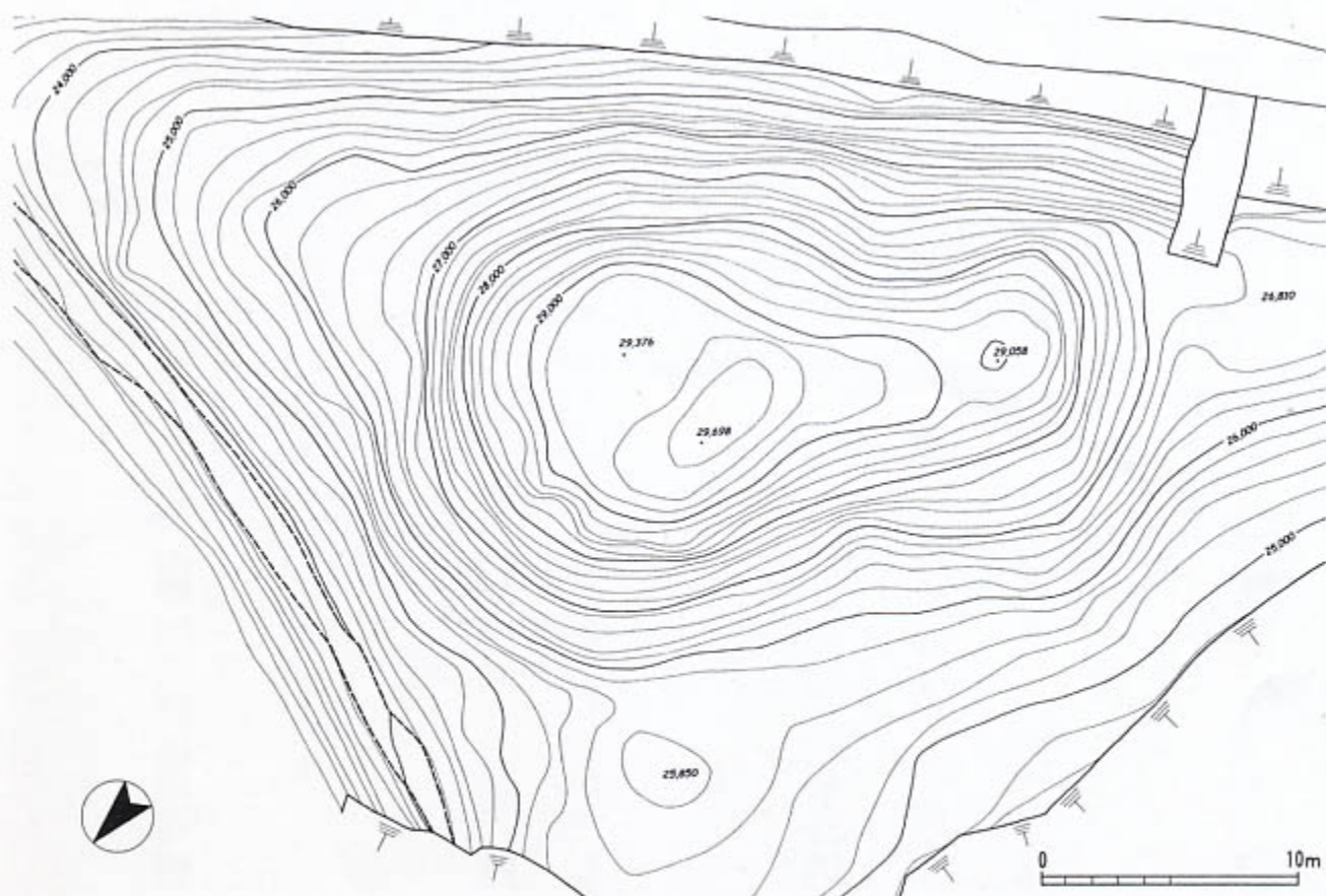
おこし古墳墳丘測量図（1：300）
