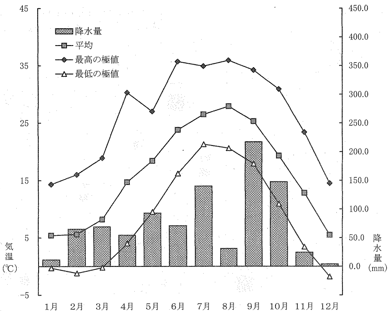
4 月別平均気温と降水量(平成17年)
