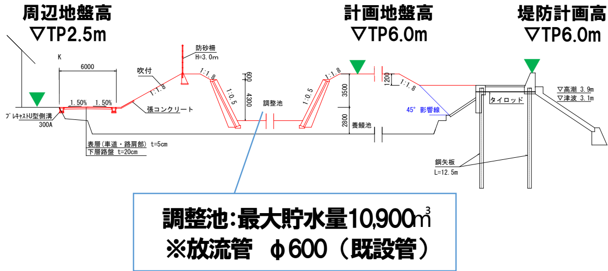
断面図 A-A'
