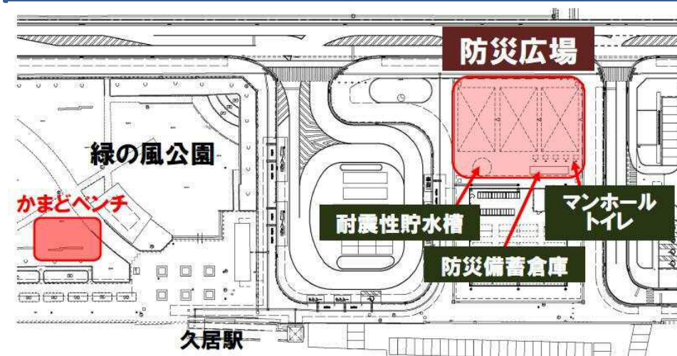
久居駅東口防災施設完成予想図
