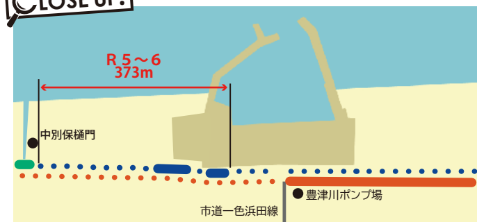
白塚漁港海岸堤防(白塚工区)
