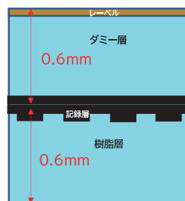
DVD盤断面図
