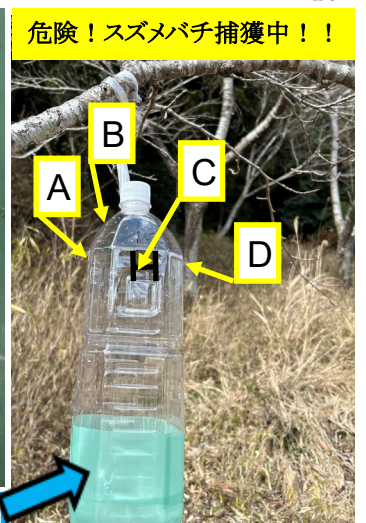
ABCDの4方向穴あけ加工
