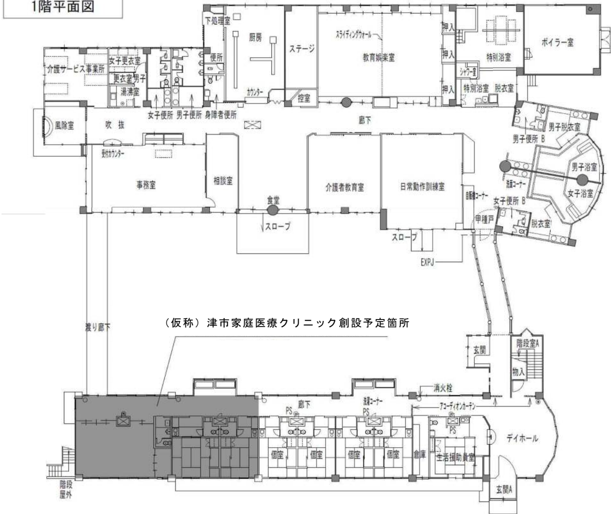
1階平面図
