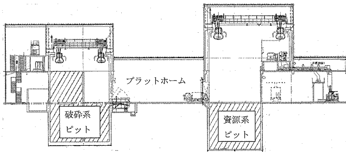
断面図
