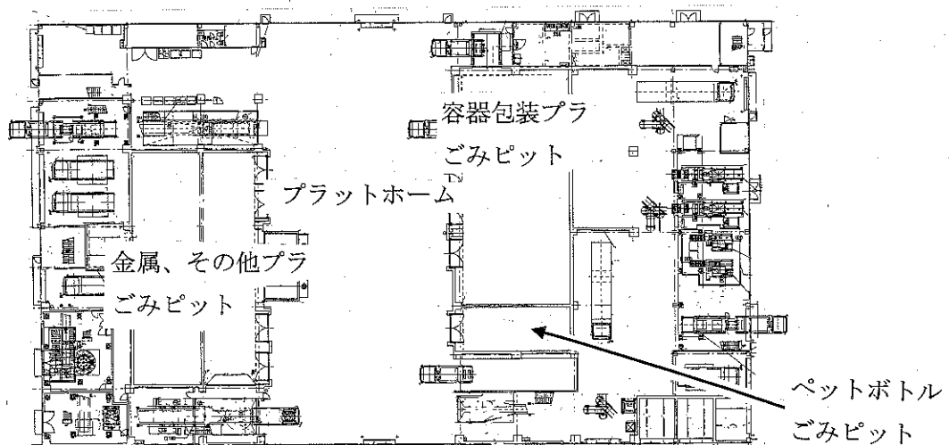
1階平面図
