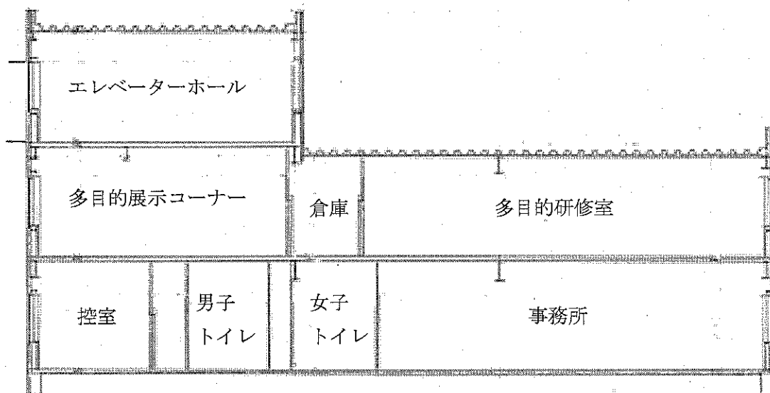
断面図
