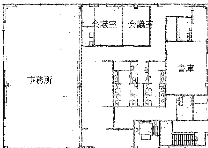
平面図 1 階
