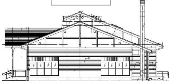
東立面図
