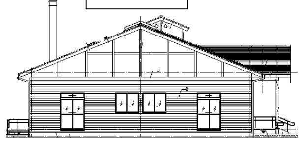
西立面図
