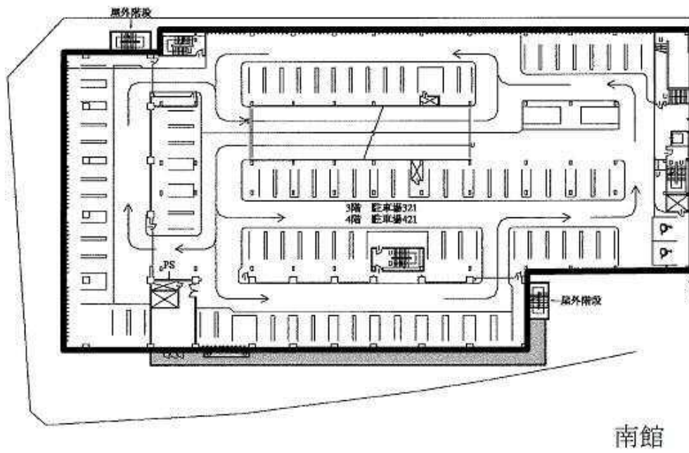
3・4階平面図
