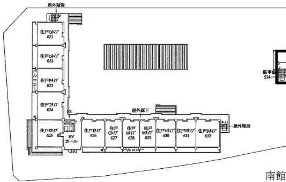
6 階平面図
