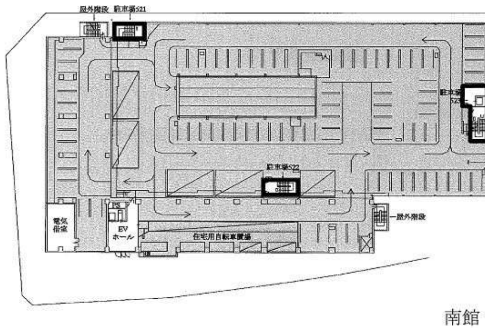
5階平面図
