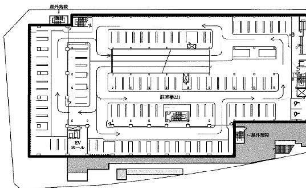
2 階平面図
