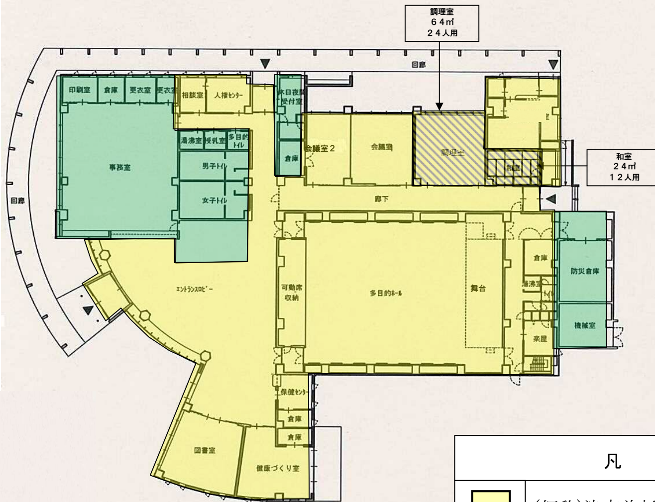
1 階平面図
