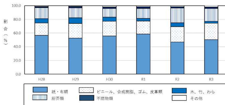
図は、津市西部クリーンセンター 可燃ごみの種類・組成の推移 (2号炉・乾ベース)
