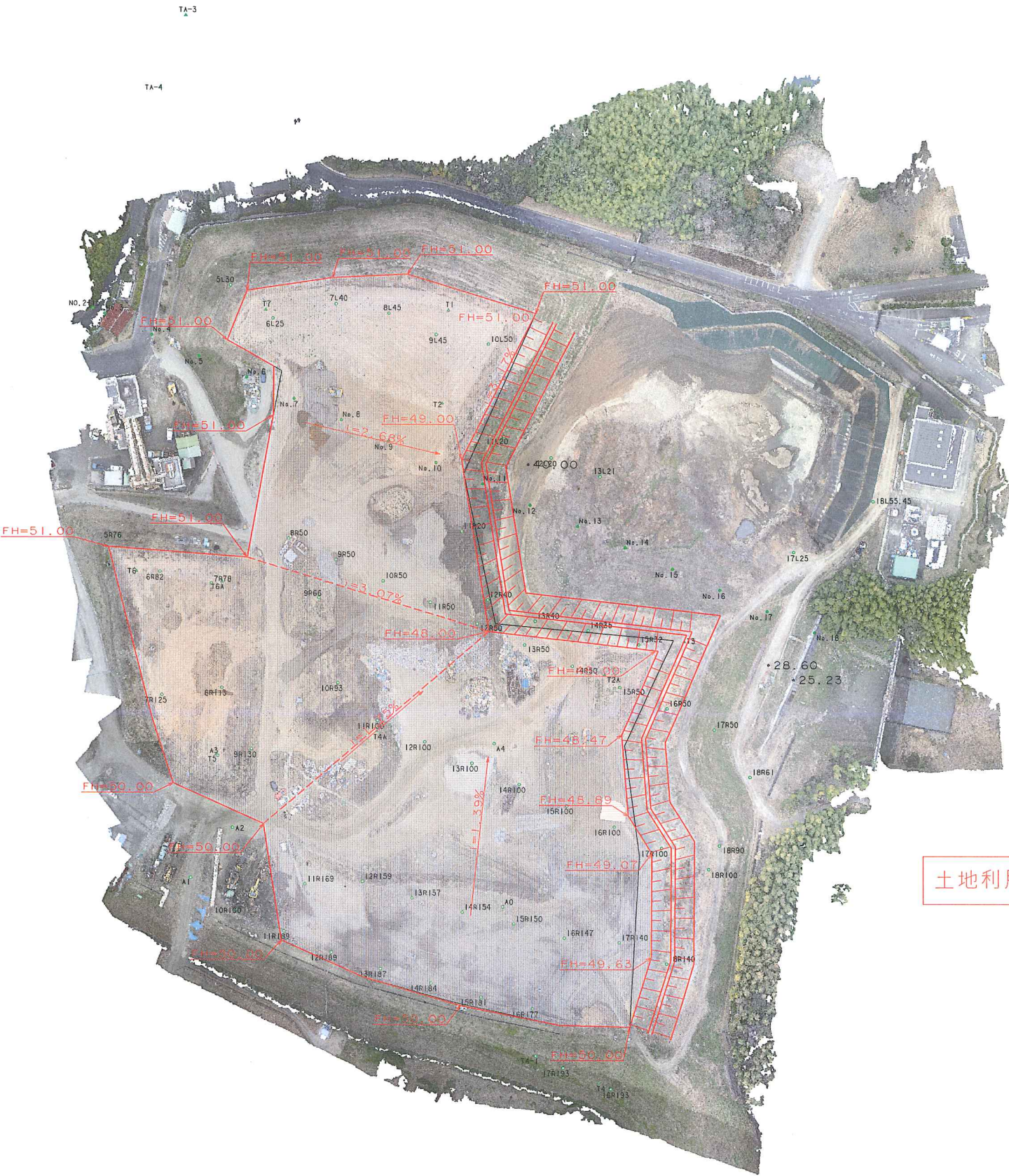
土地利用計画平面図
