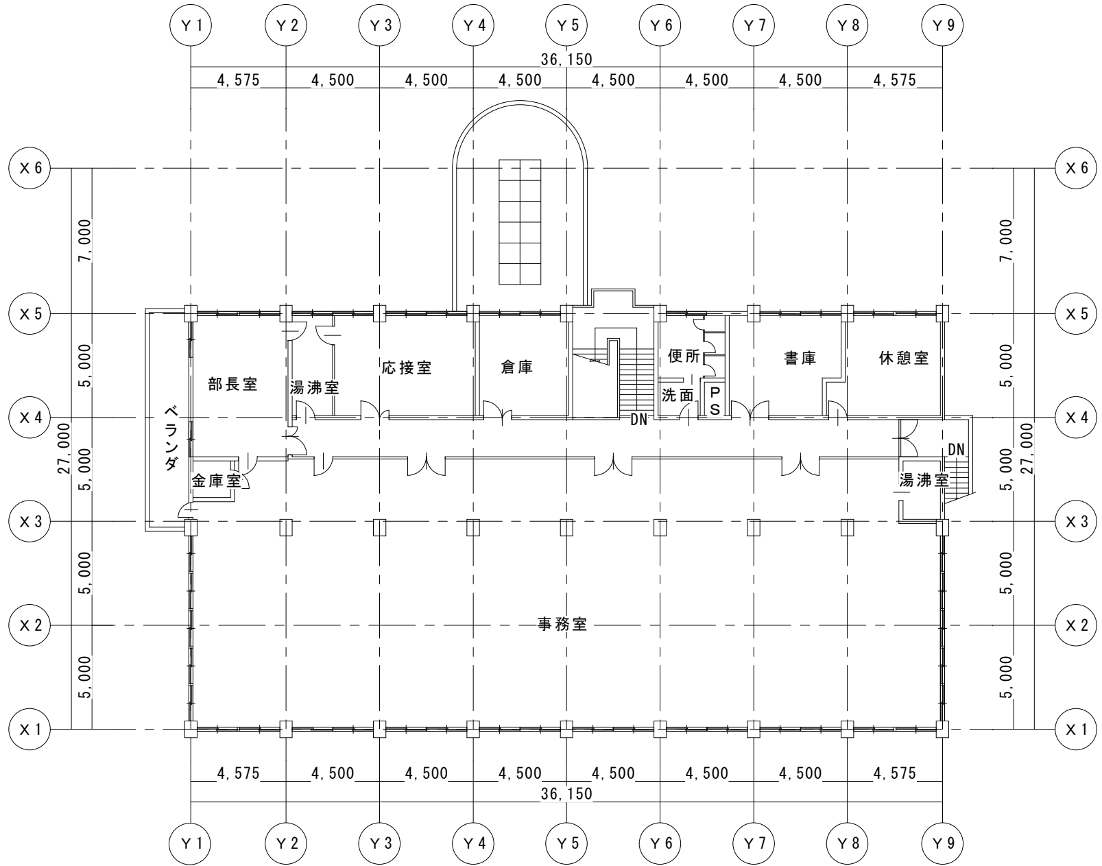
2 階平面図
