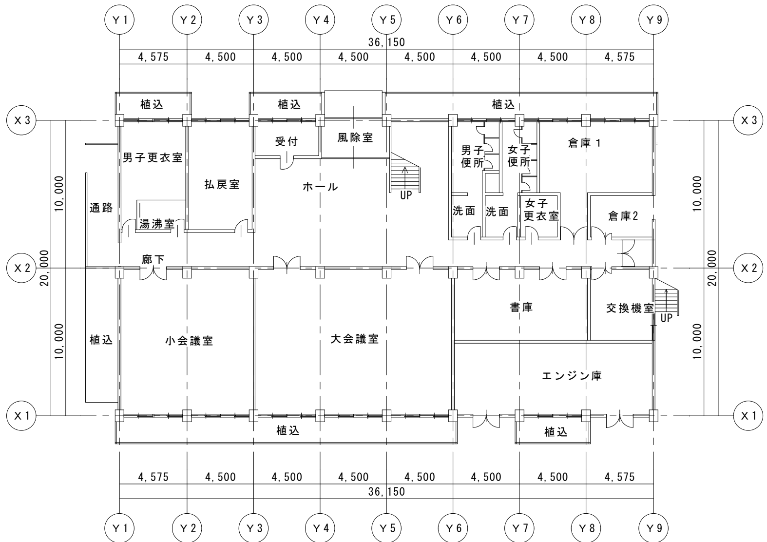
1 階平面図
