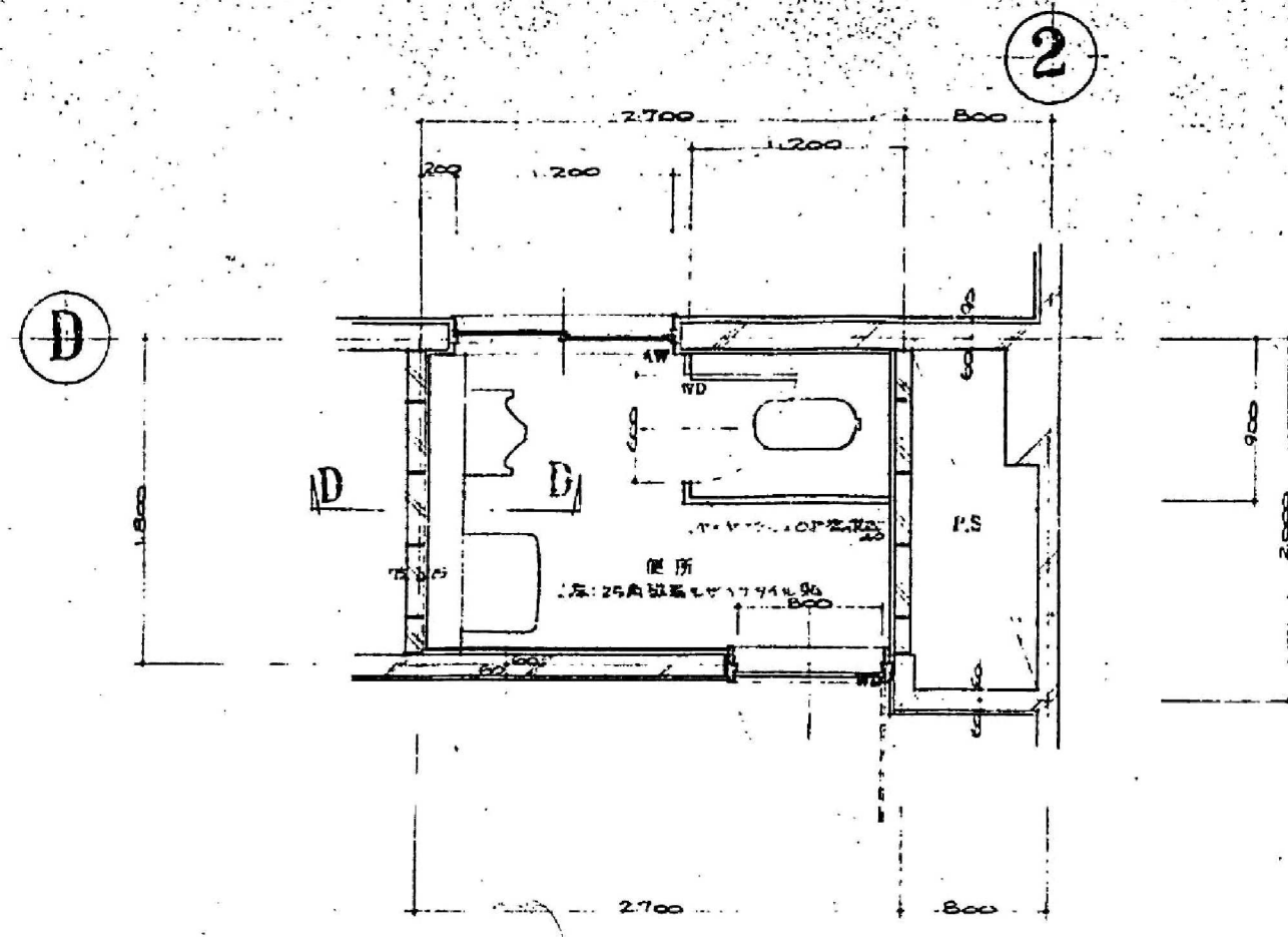
1 階正平面詳細図 S=1/42
