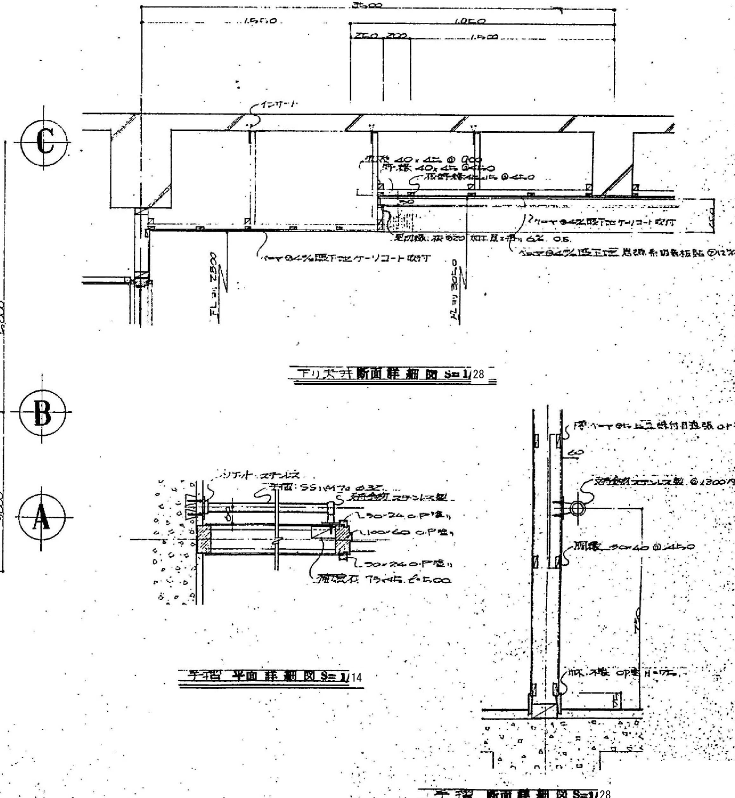
下り大式断面詳細図 S=1/28
