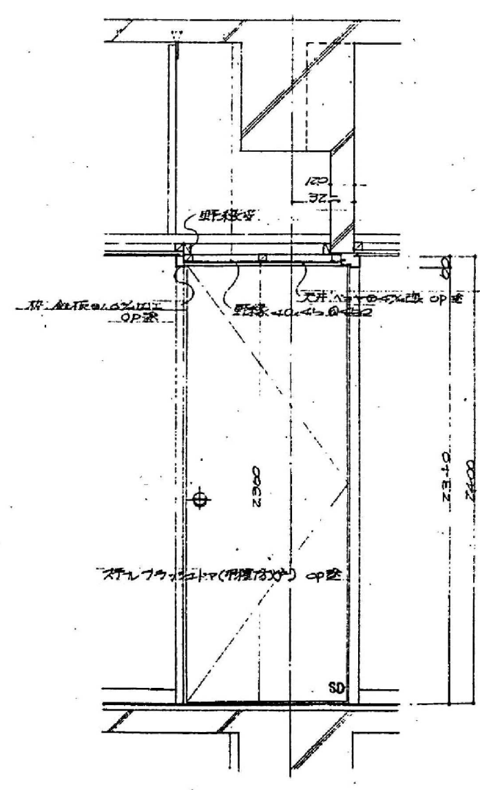
断面C-C詳細図 S=1/28
