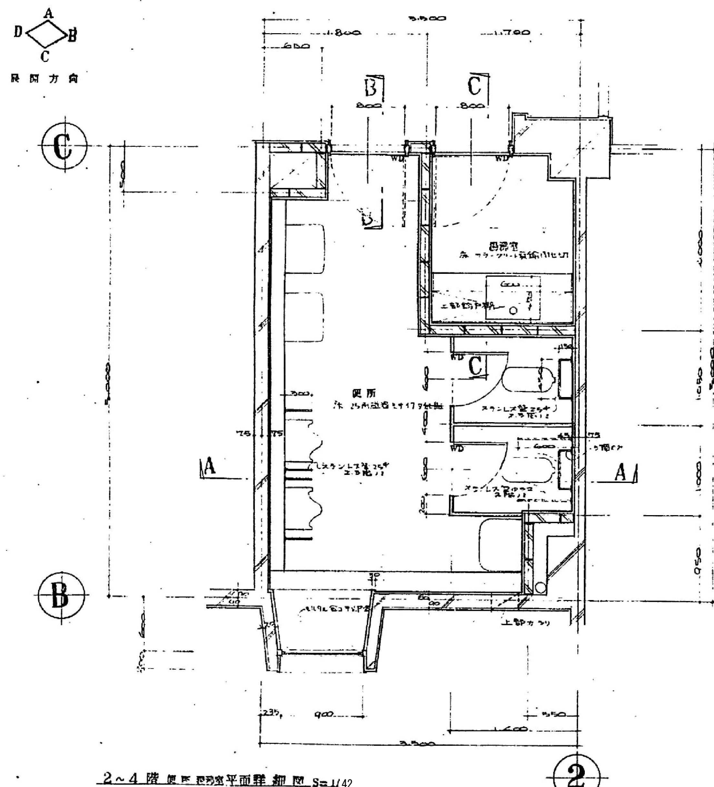
2~4 階 便所 和 浴室 平面 詳細 図 S=1/42
