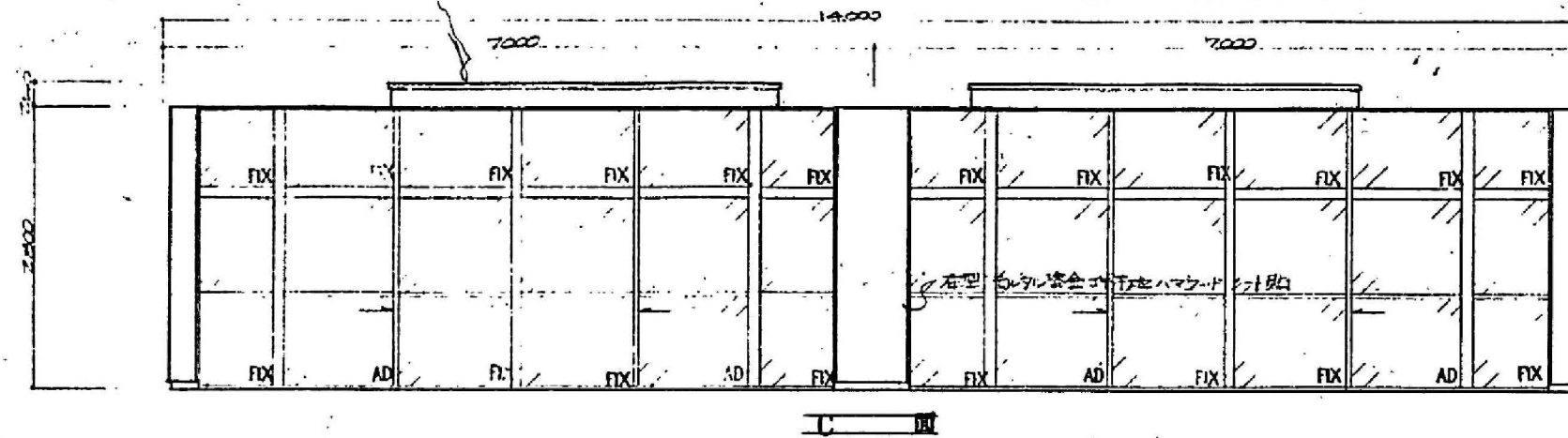
大会議室 立面図 S=1/70
