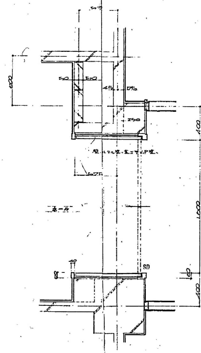
断面B-B詳細図 S=1/28
