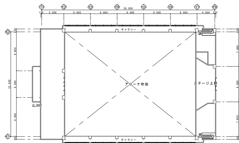
2階平面図
