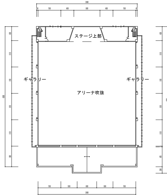
2階平面図
