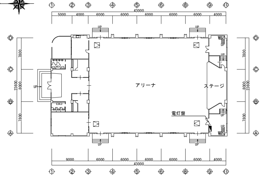
1階平面図
