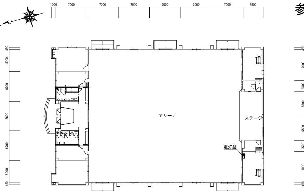
1階平面図
