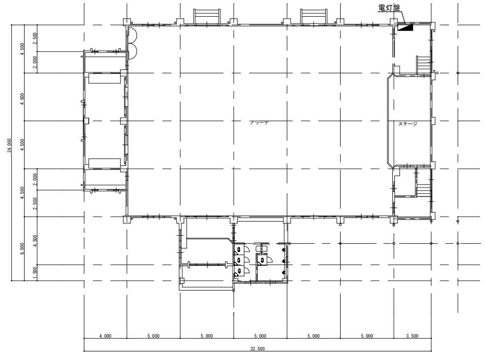
1階平面図
