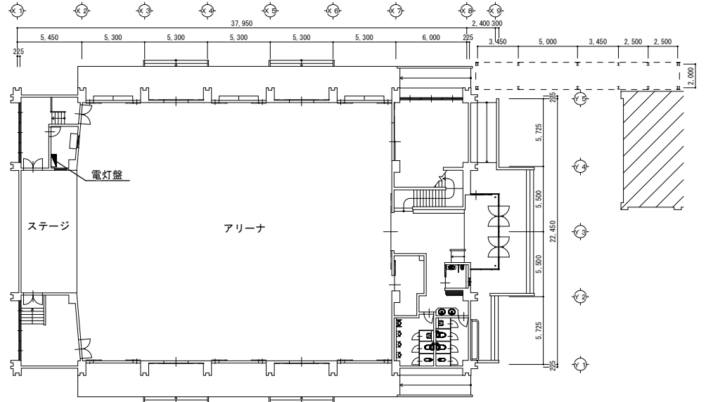
1階平面図
