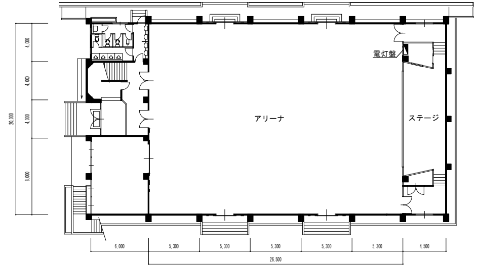
1階平面図
