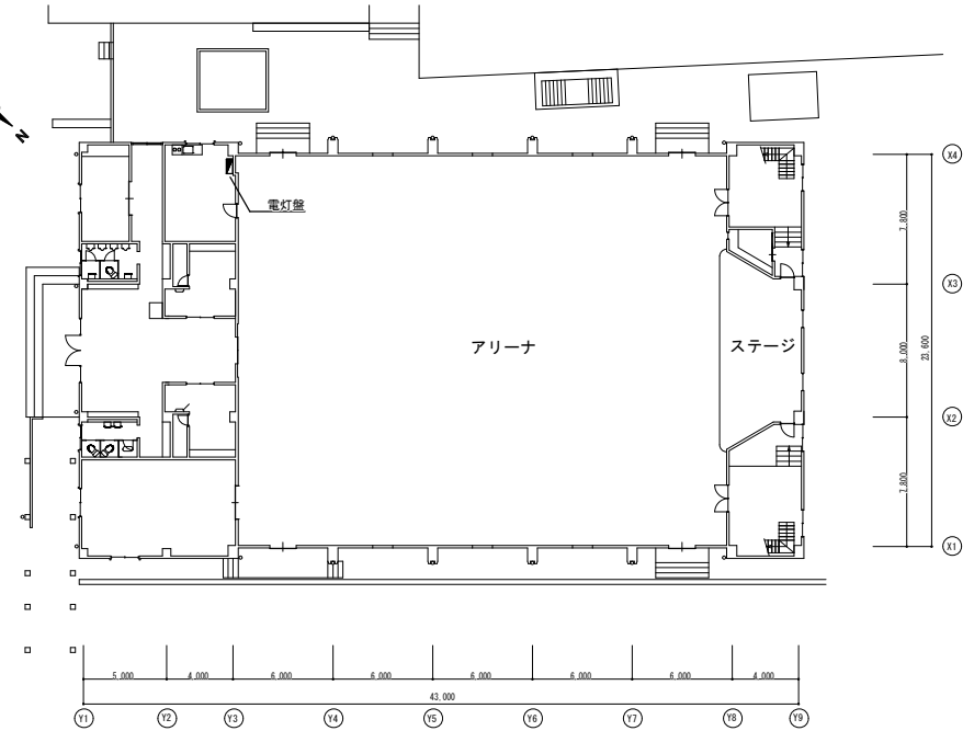
1階平面図
