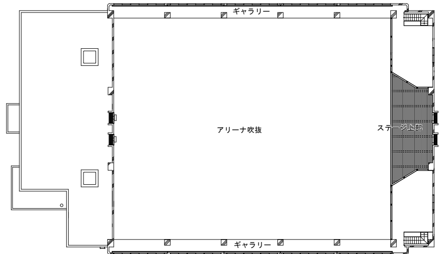
2階平面図
