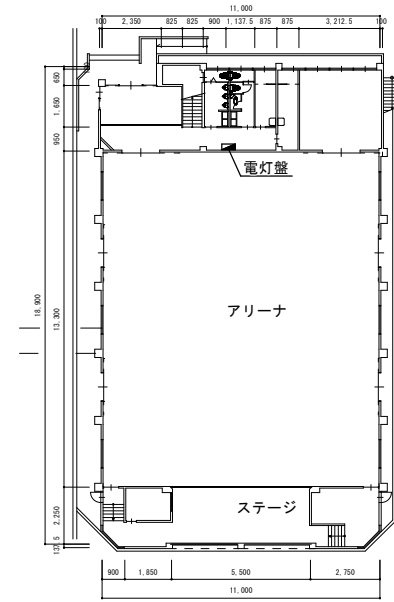
1階平面図
