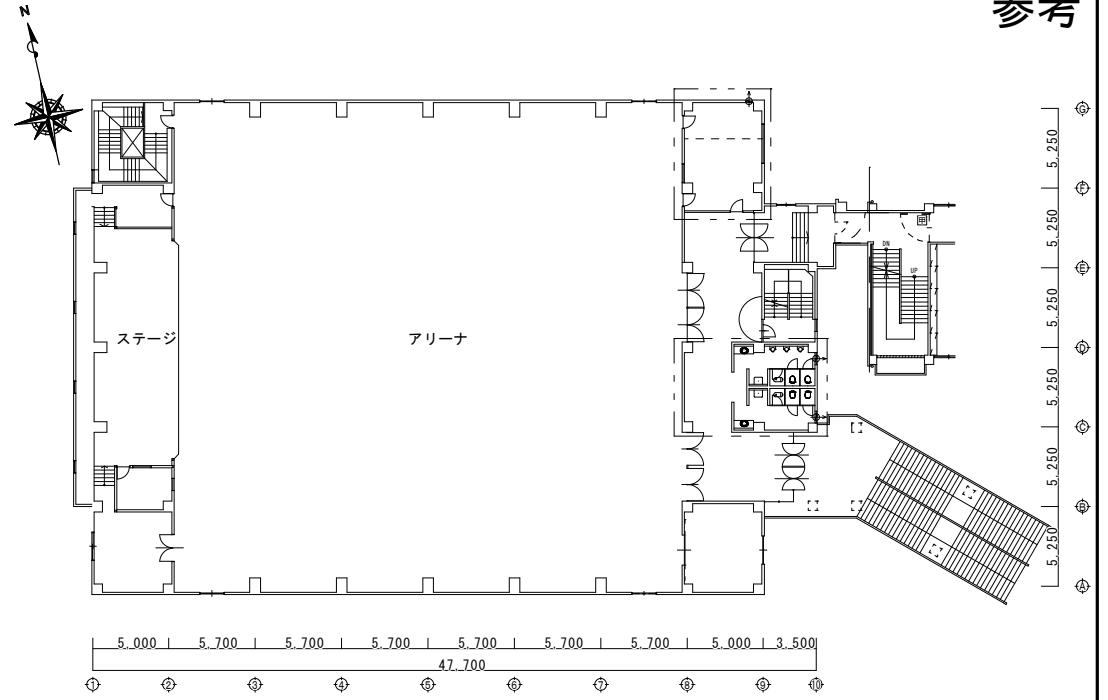
2階平面図
