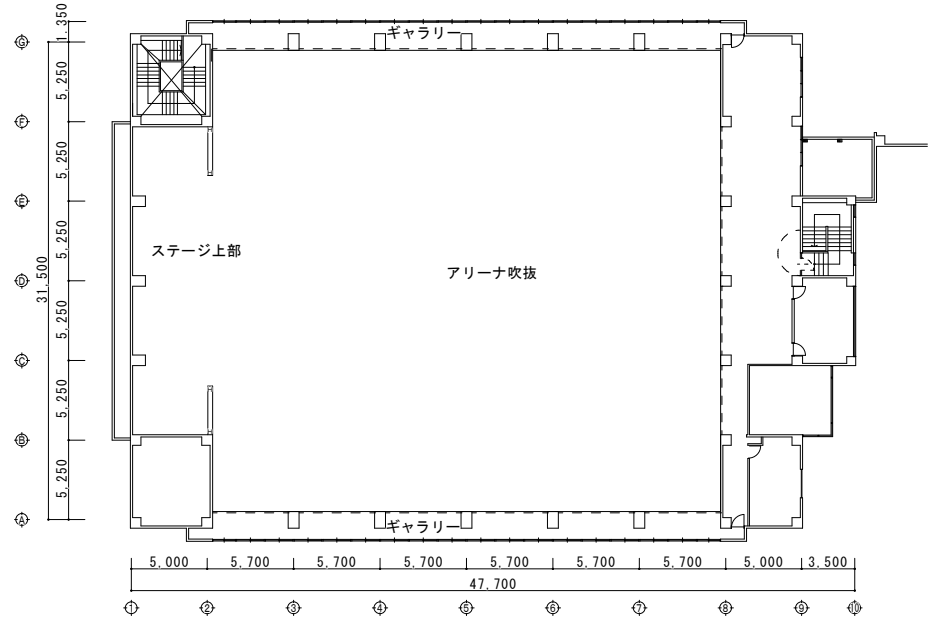
3階平面図
