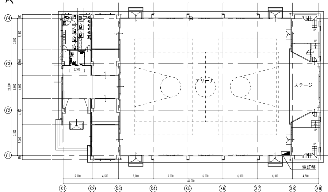
1階平面図
