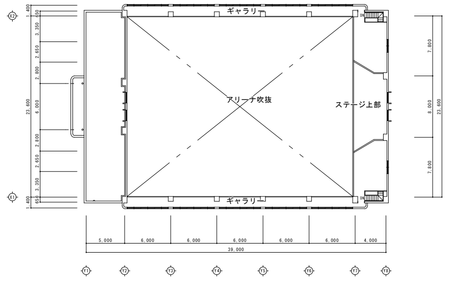
2階平面図
