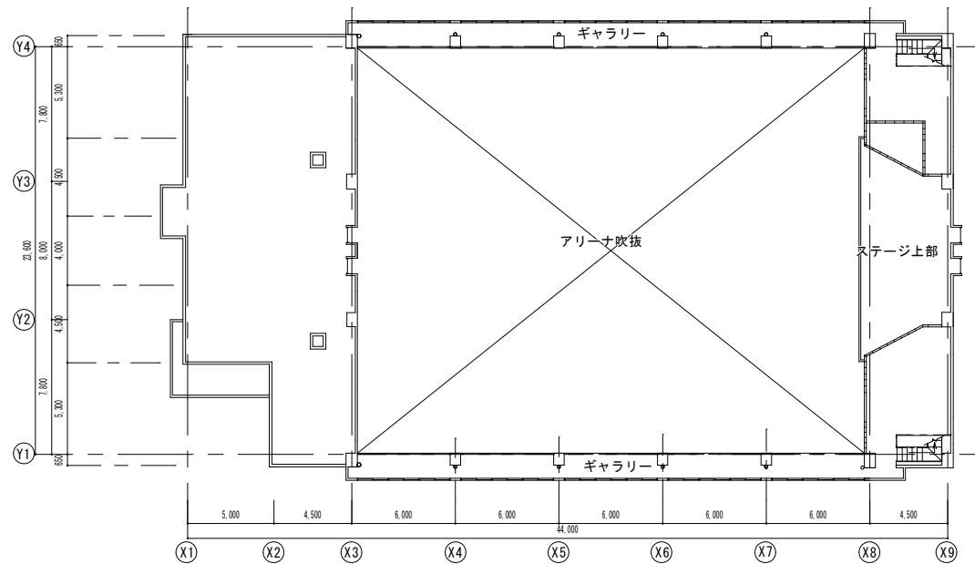
2階平面図
