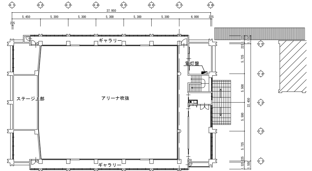
2階平面図
