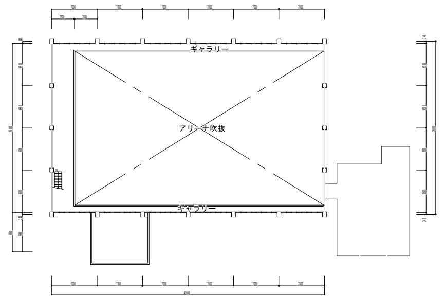
2階平面図
