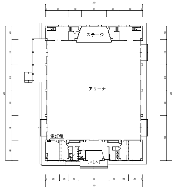
1階平面図
