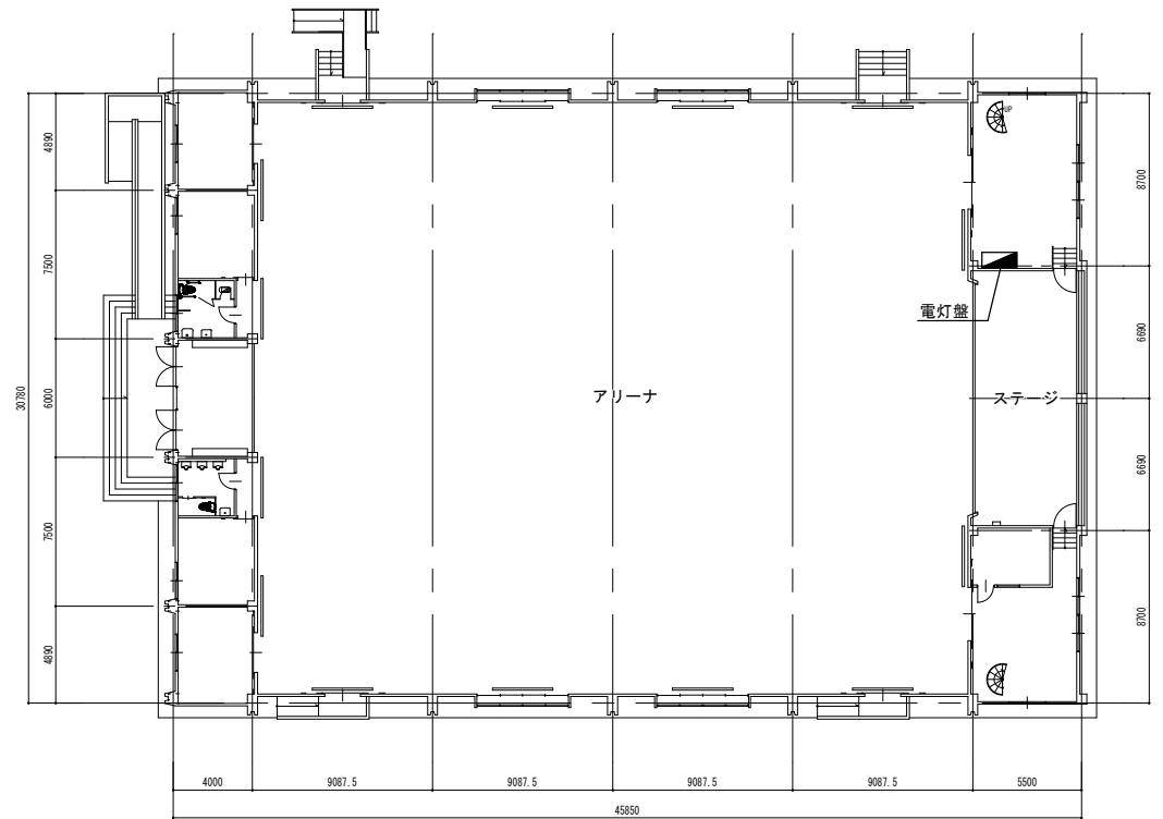
1階平面図
