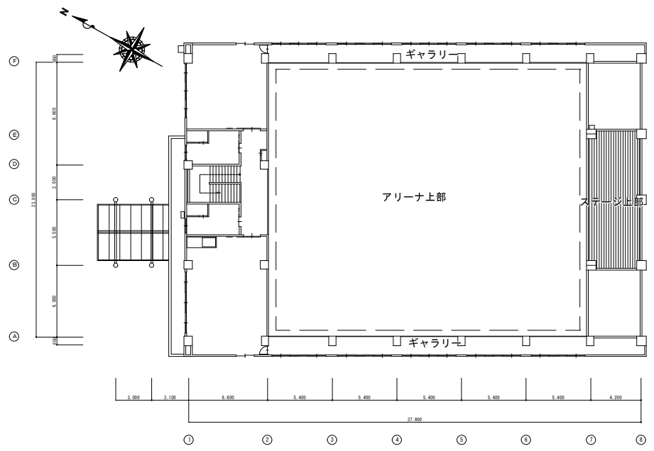
2階平面図
