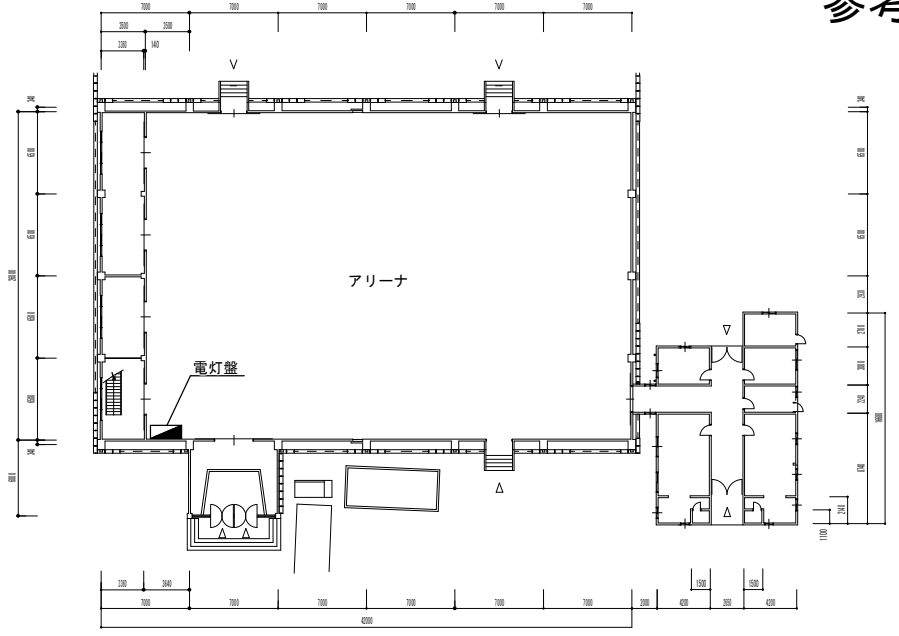
1階平面図
