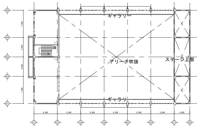
2階平面図
