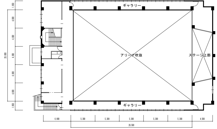
2階平面図
