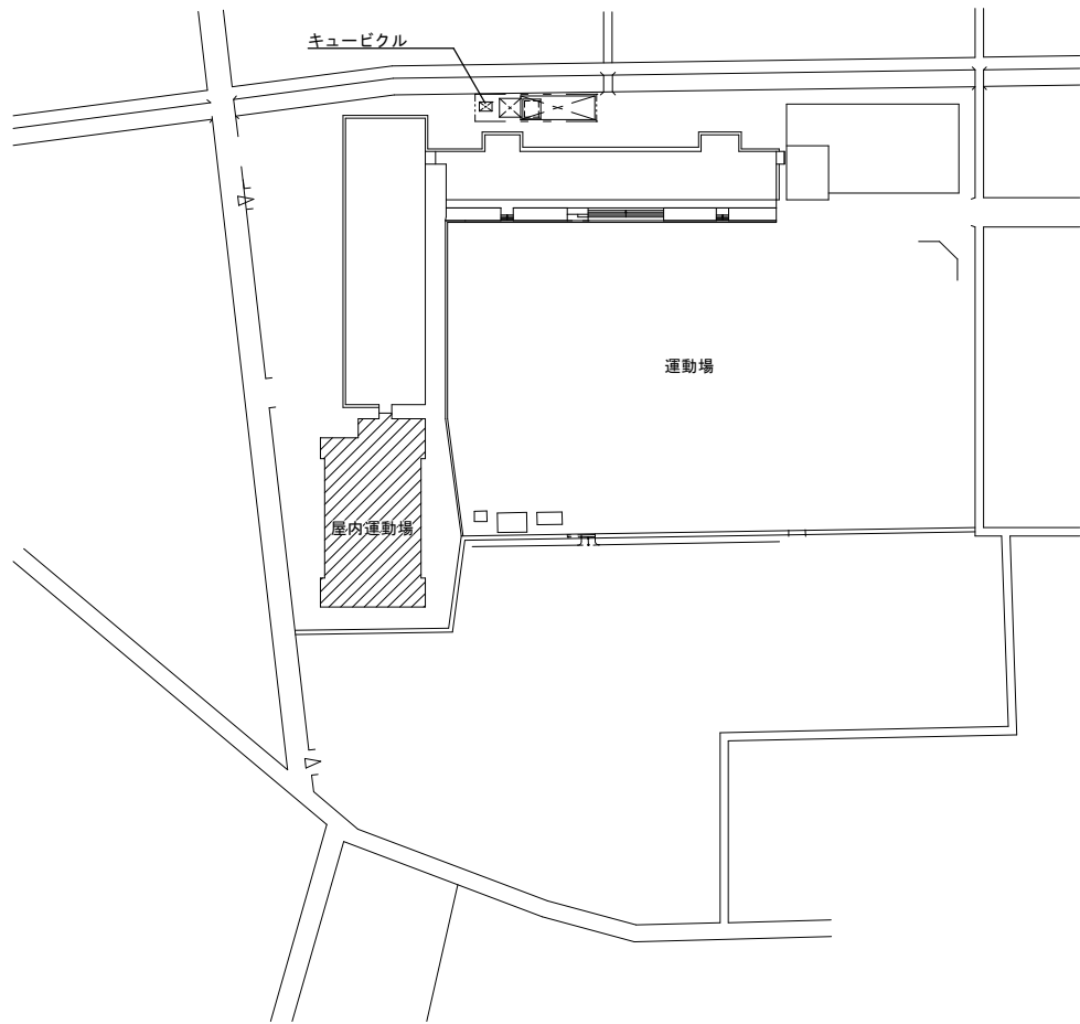
配置図
