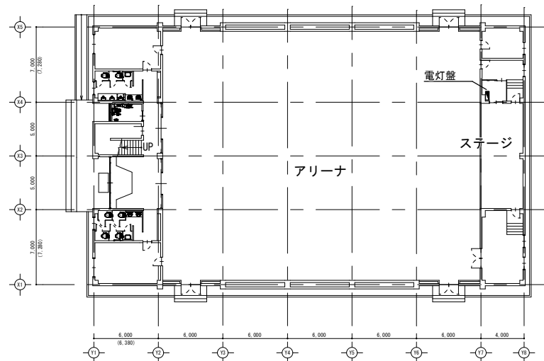
1階平面図
