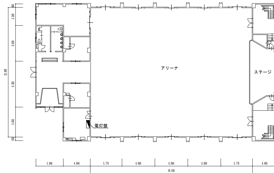
1階平面図
