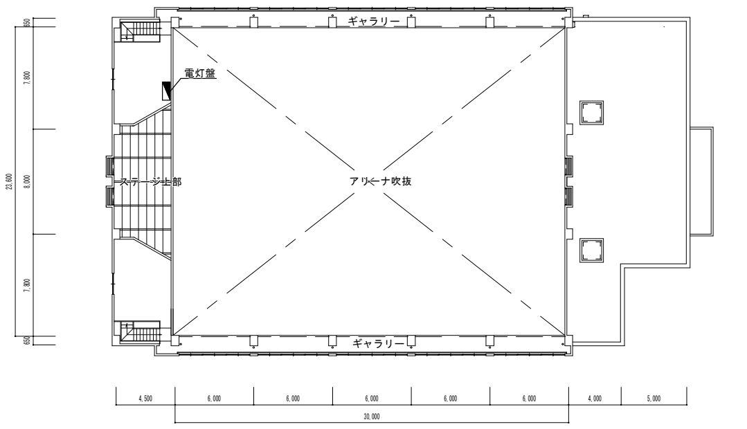
2階平面図
