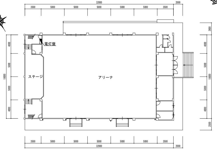
1階平面図
