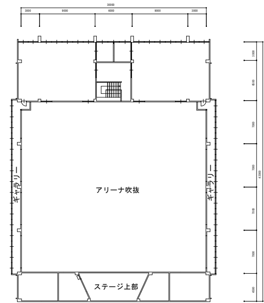
2階平面図
