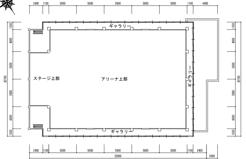
2階平面図
