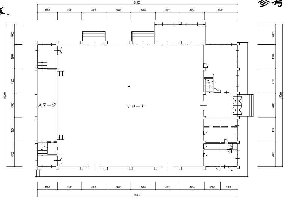
1階平面図
