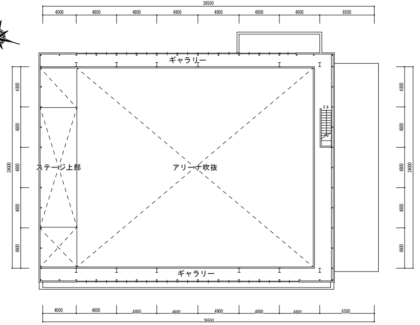
2階平面図
