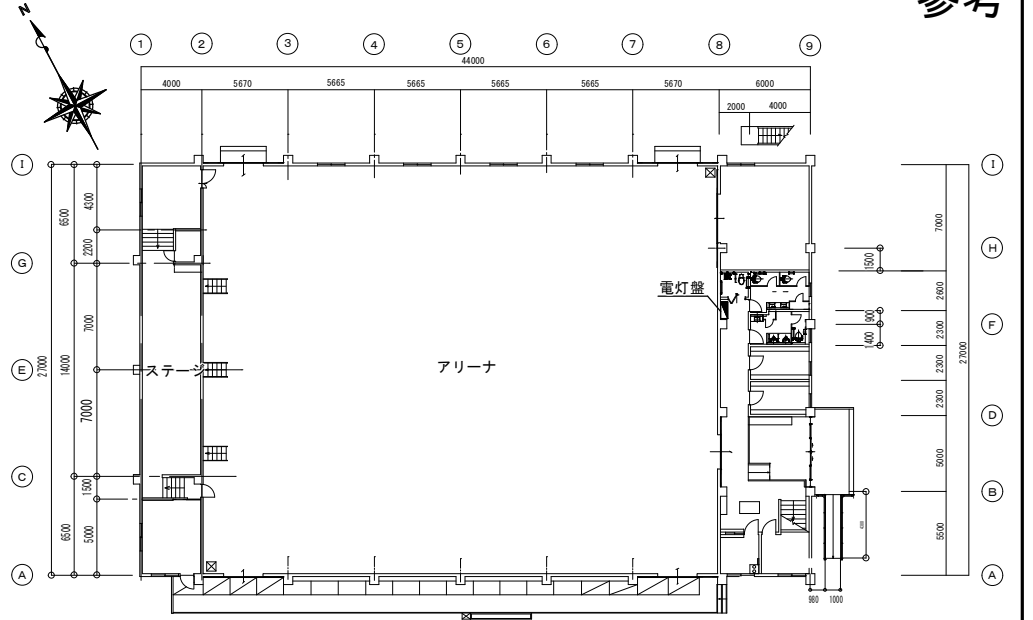
1階平面図
