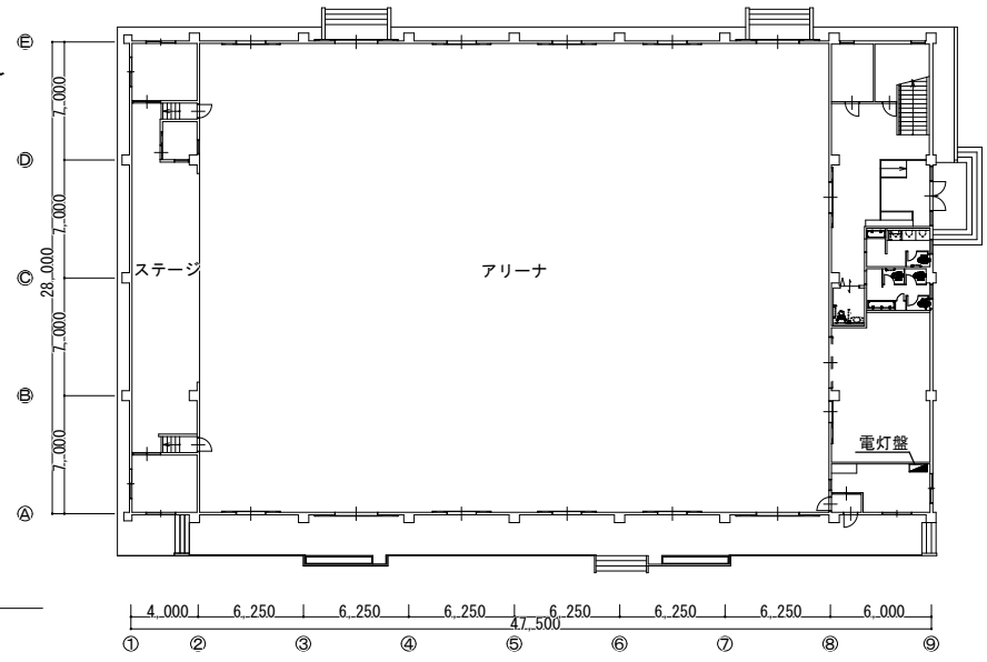
1階平面図
