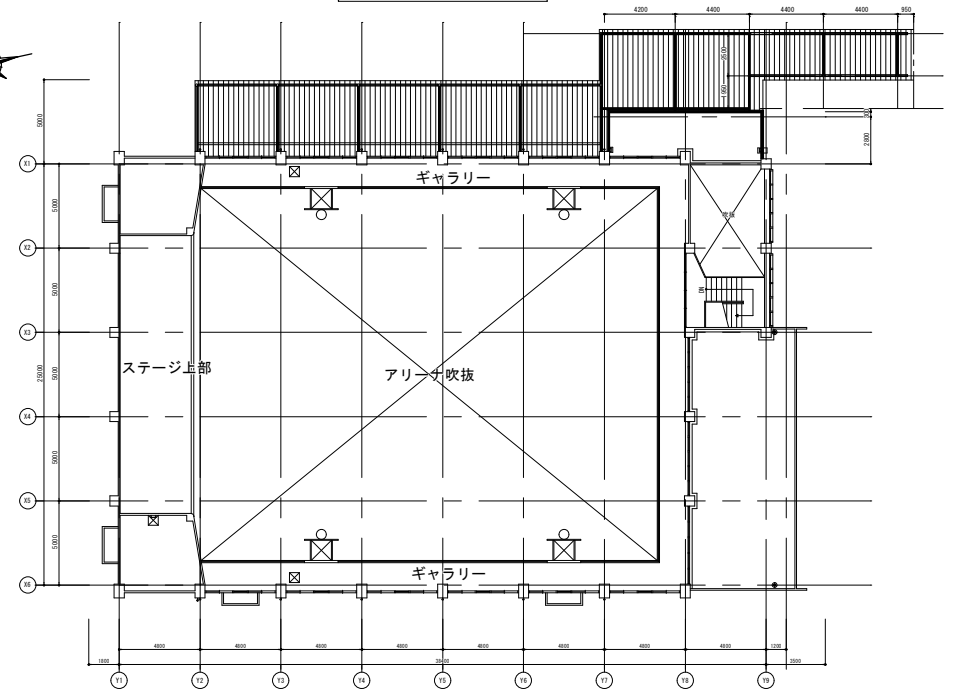
2階平面図
