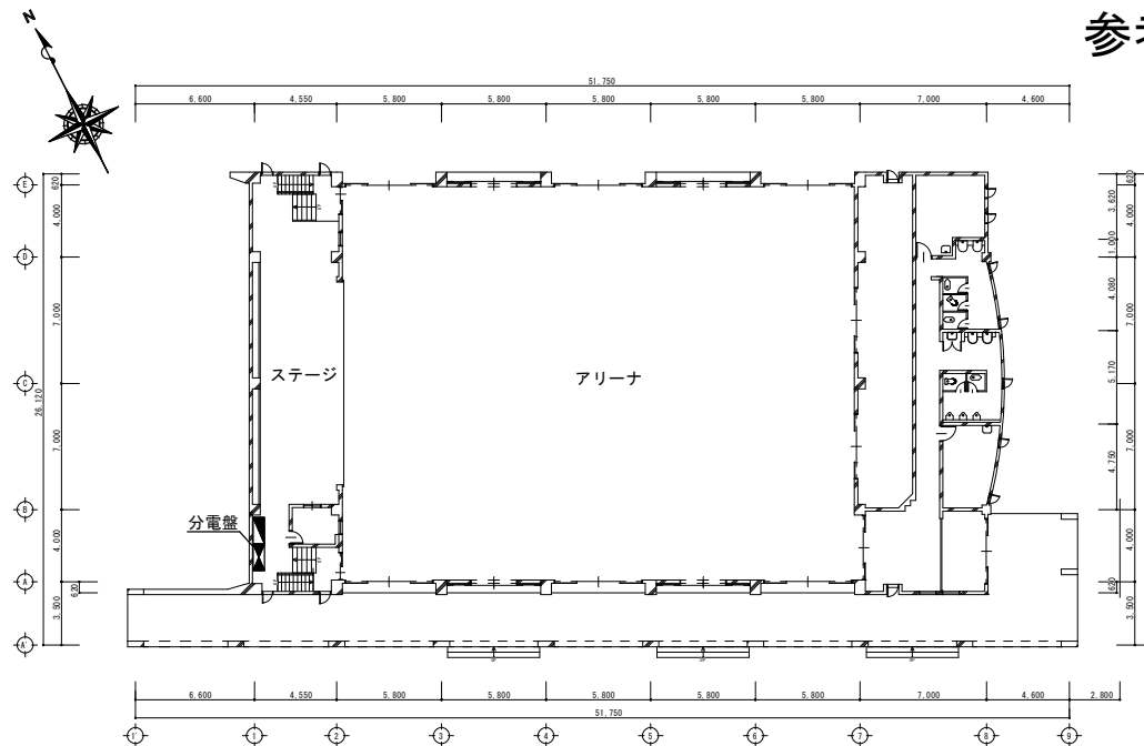
1階平面図
