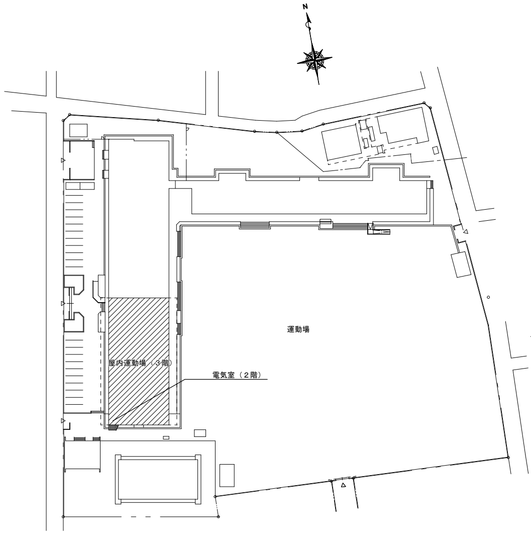
配置図
