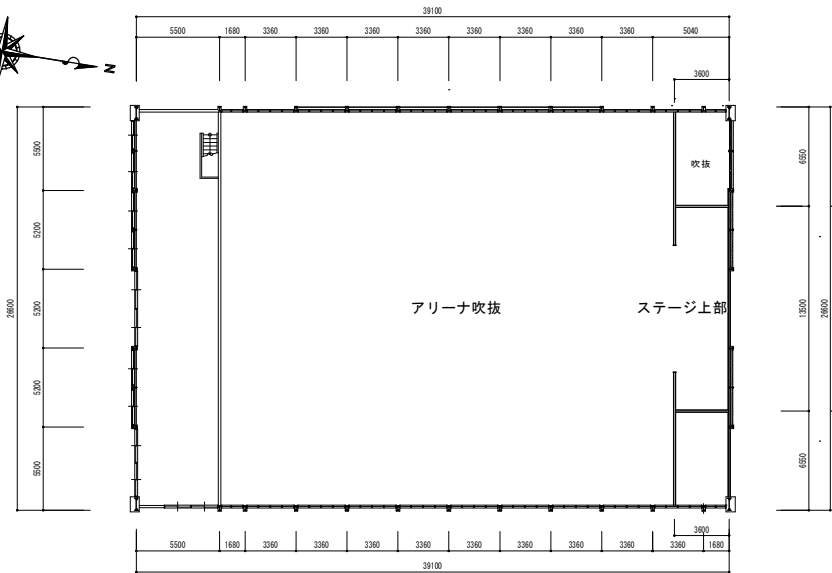
2階平面図
