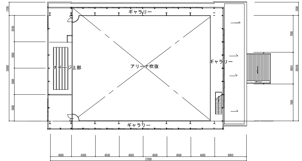
2階平面図
