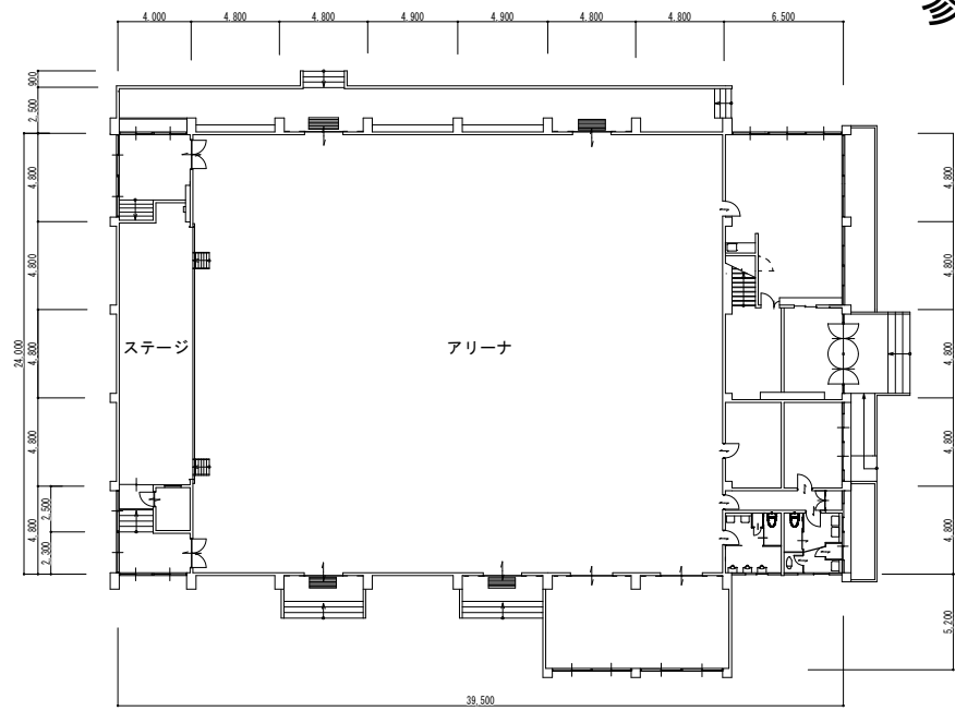
1階平面図
