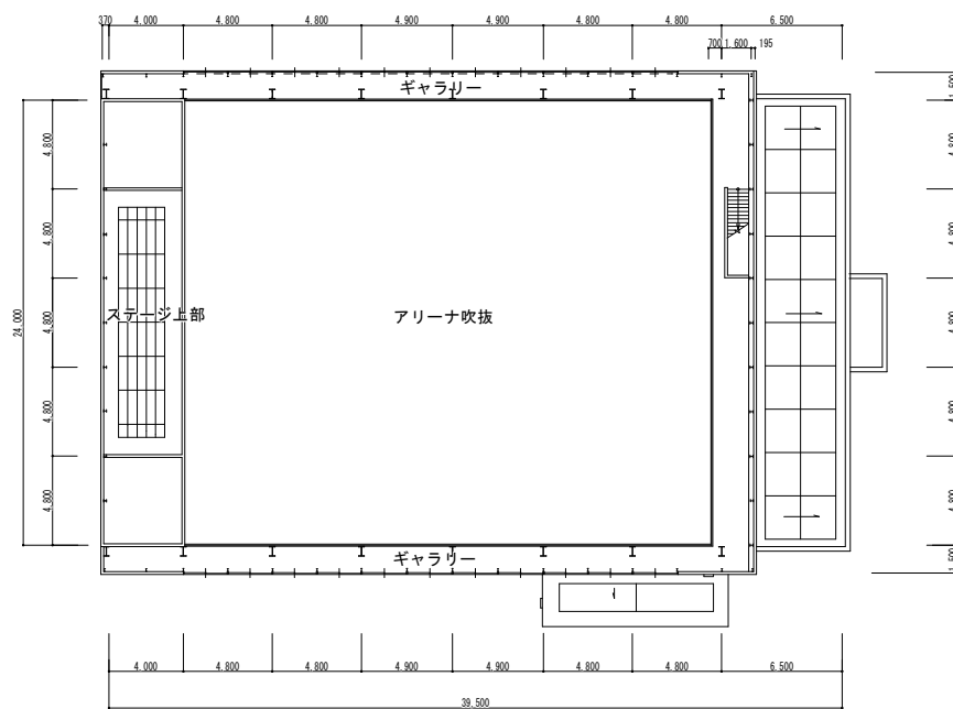
2階平面図
