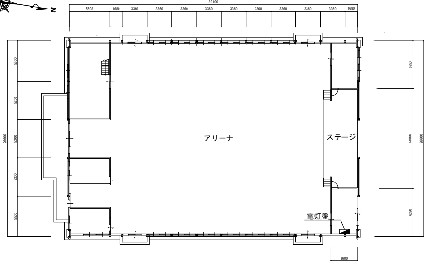
1階平面図
