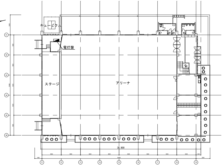
1階平面図
