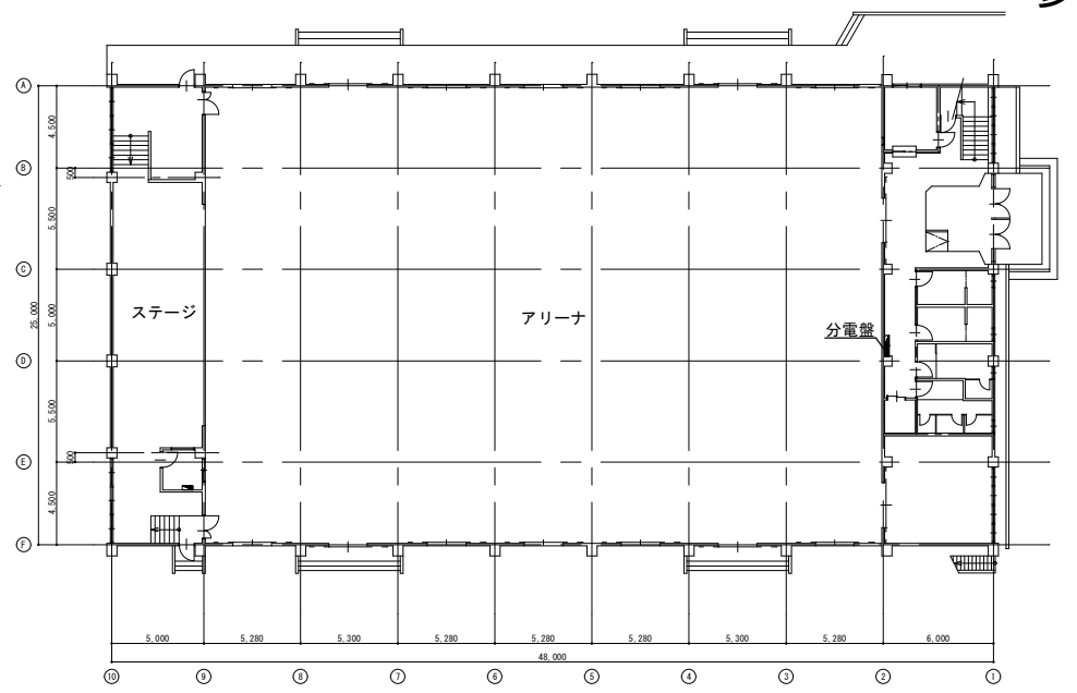
1階平面図
