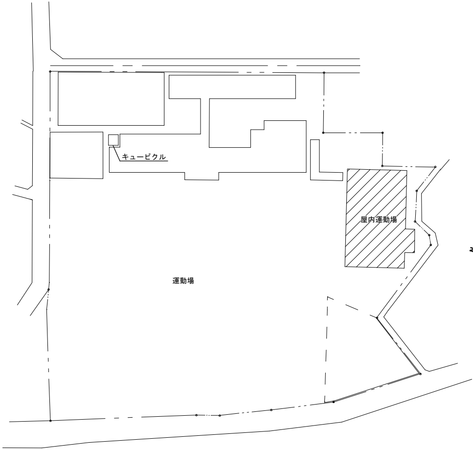
配置図
