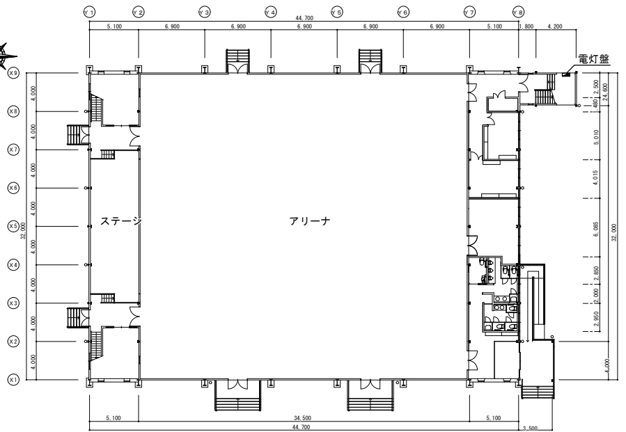
1階平面図
