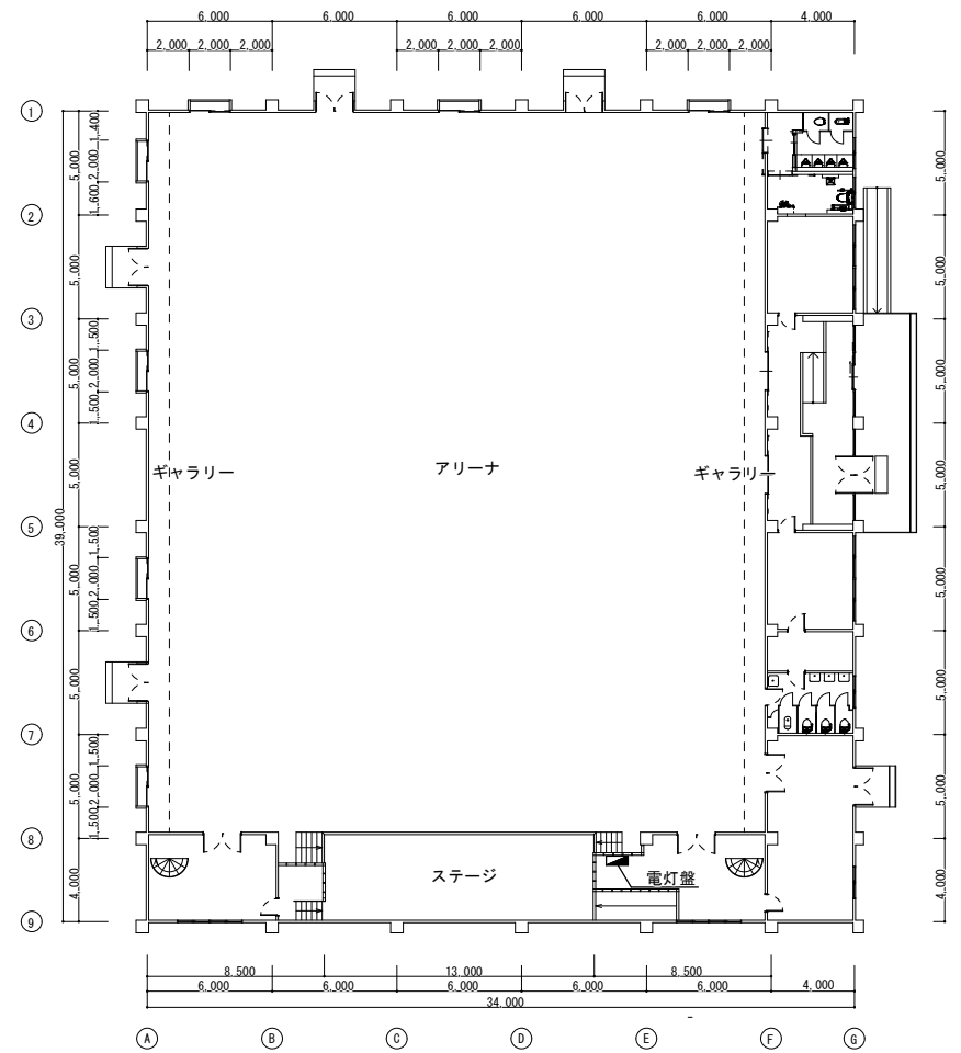
1階平面図
