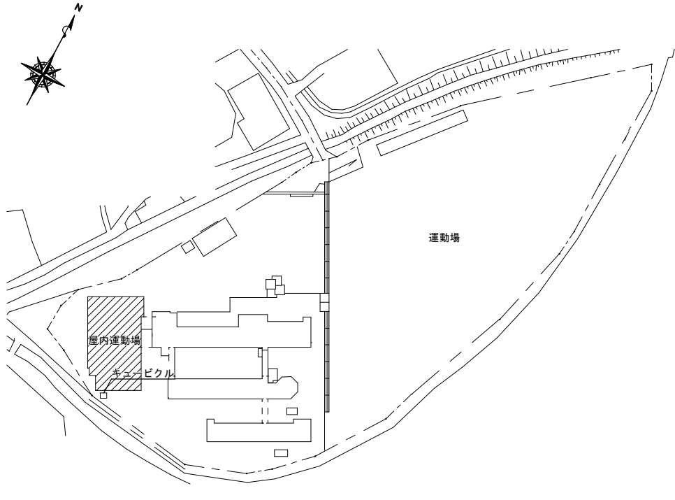
配置図
