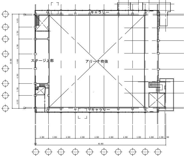
2階平面図
