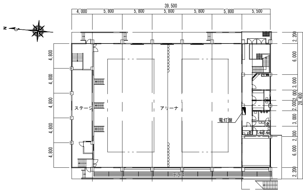
1階平面図
