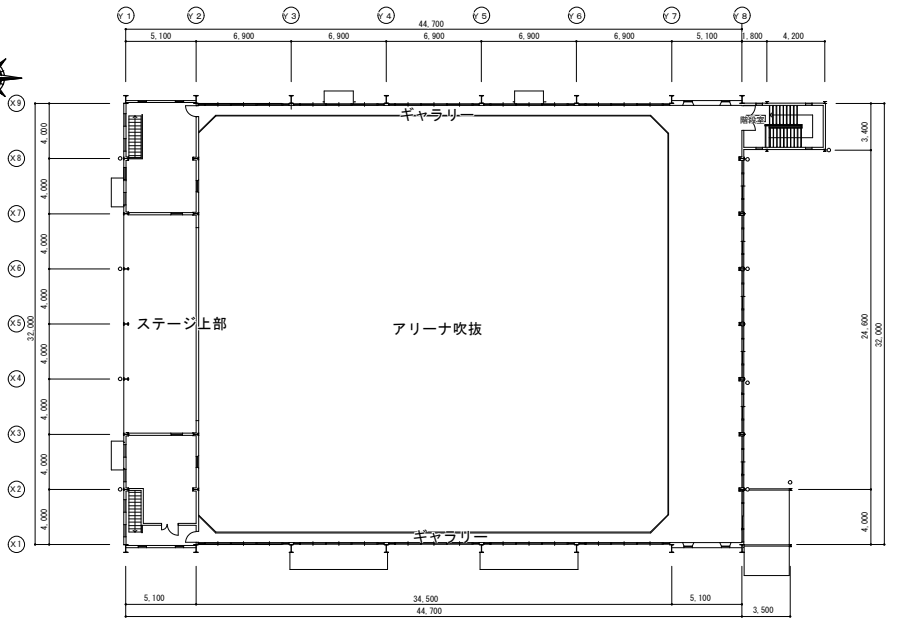
2階平面図
