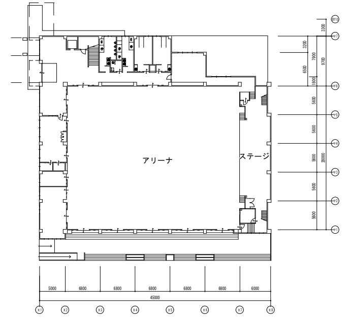
1階平面図
