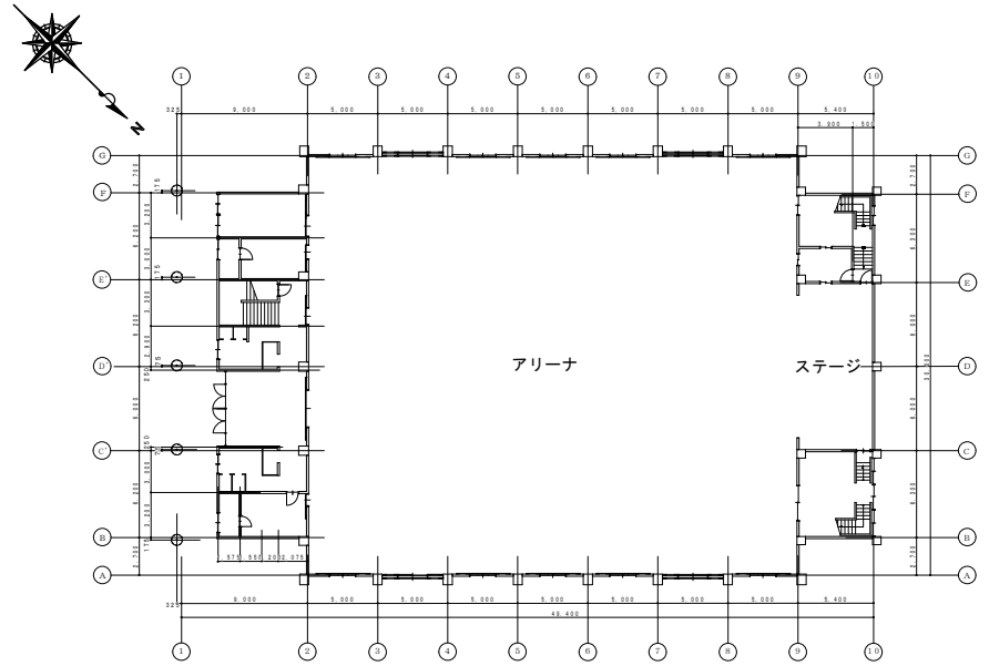
1階平面図
