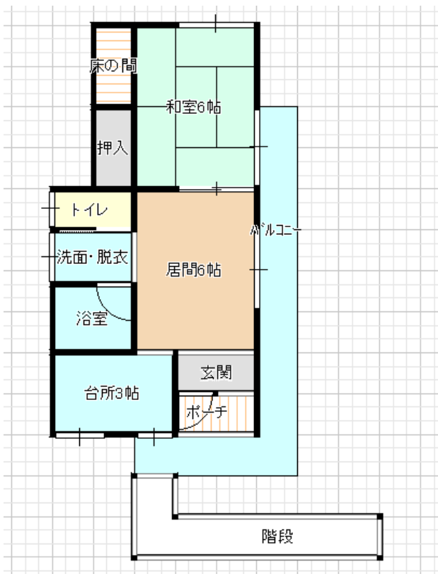
間取図
