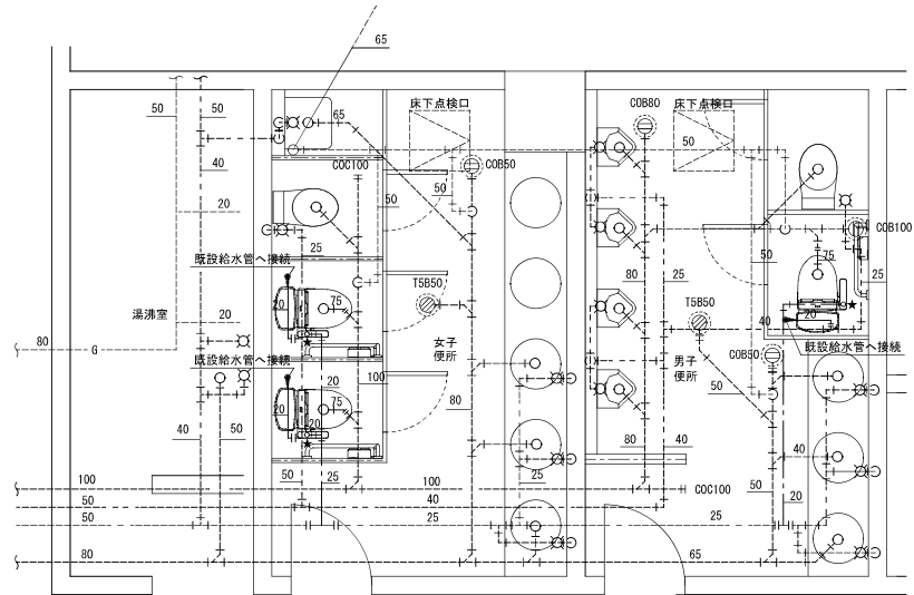
1階③平面詳細図（改修後） S=1/40
