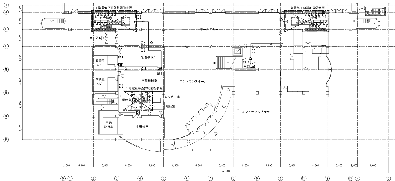
1階平面図 S=1/300
