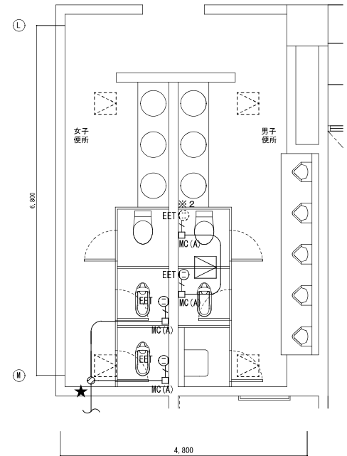
2階平面詳細図 S=1/50
