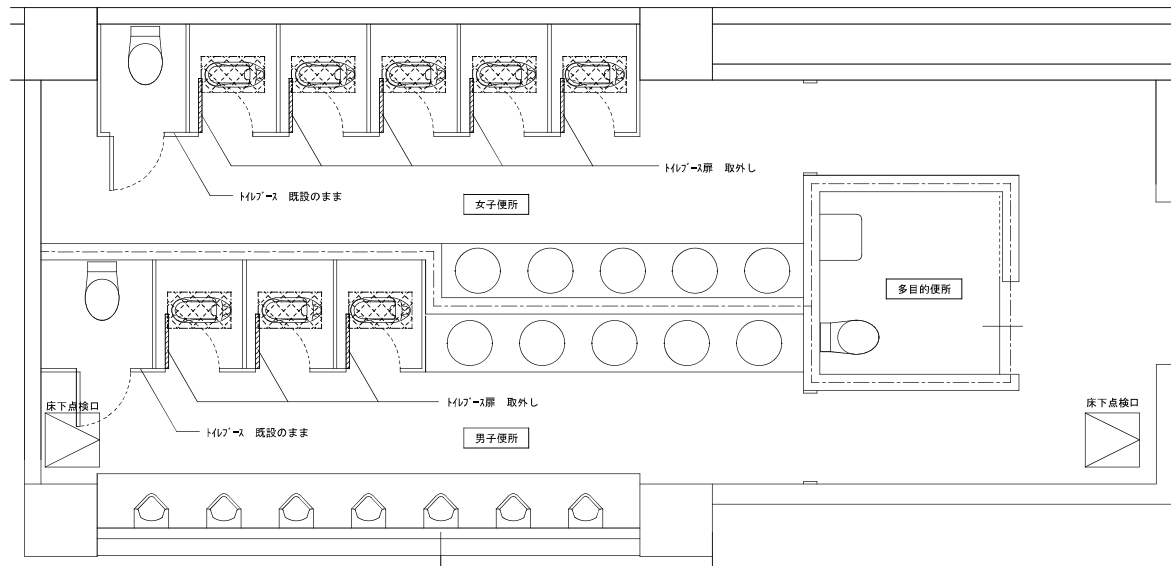
1階①平面詳細図（改修前） S=1/40
