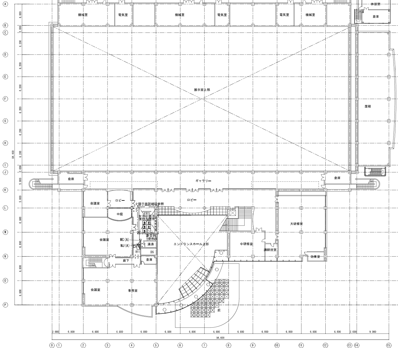
2階平面図 1/300
