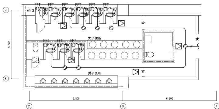
1階 平面詳細図① S=1/80
