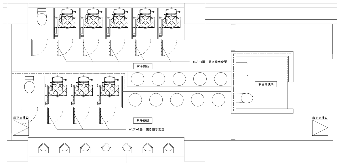
1階①平面詳細図（改修後） S=1/40
