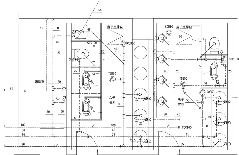
1階③平面詳細図（改修前） S=1/40
