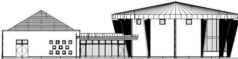
(南側)
