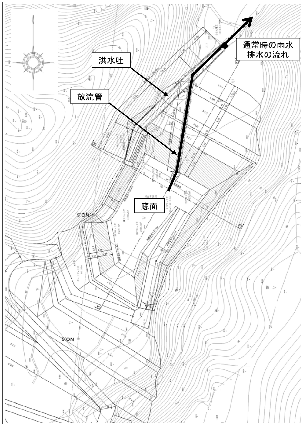
図 3.3.4-15 防災調整池平面図
