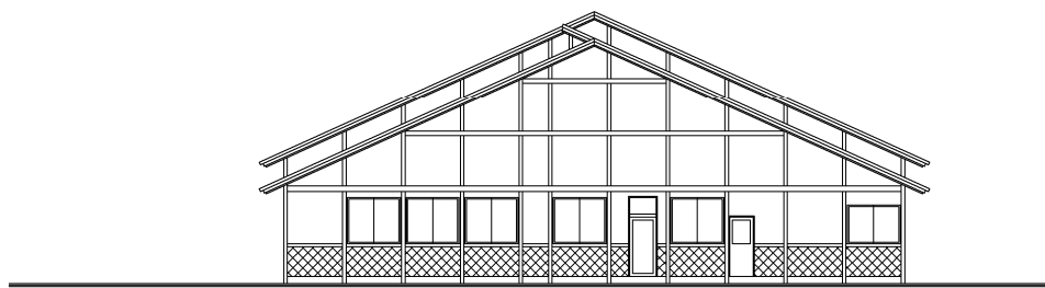
図 3.3.4-9 管理棟概略東立面図
