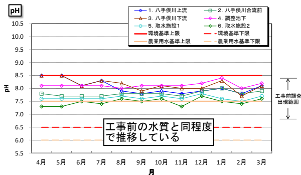
水質結果変動【 pH 】
