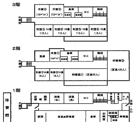
●本館配置図
