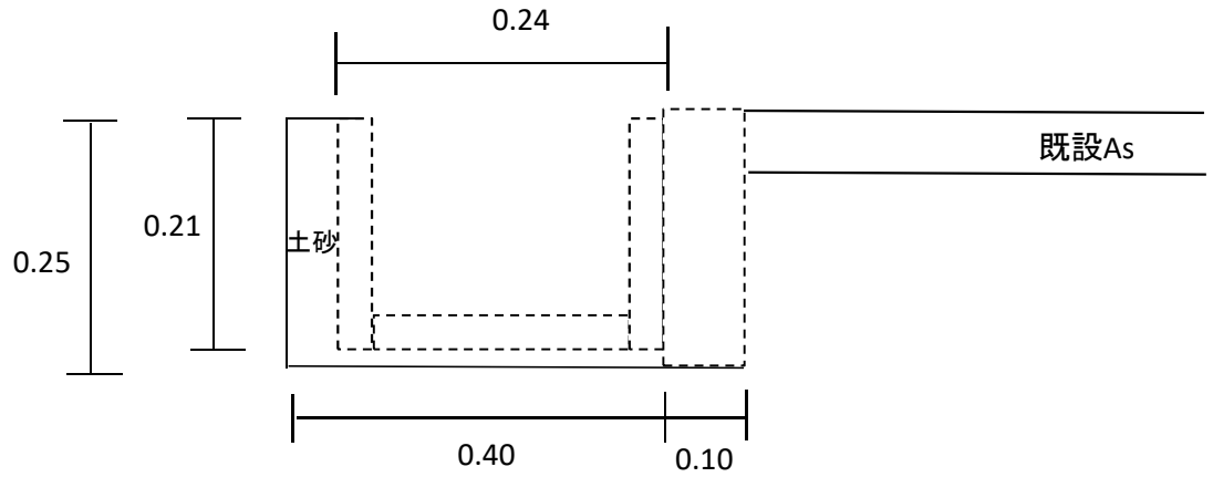
断面図
