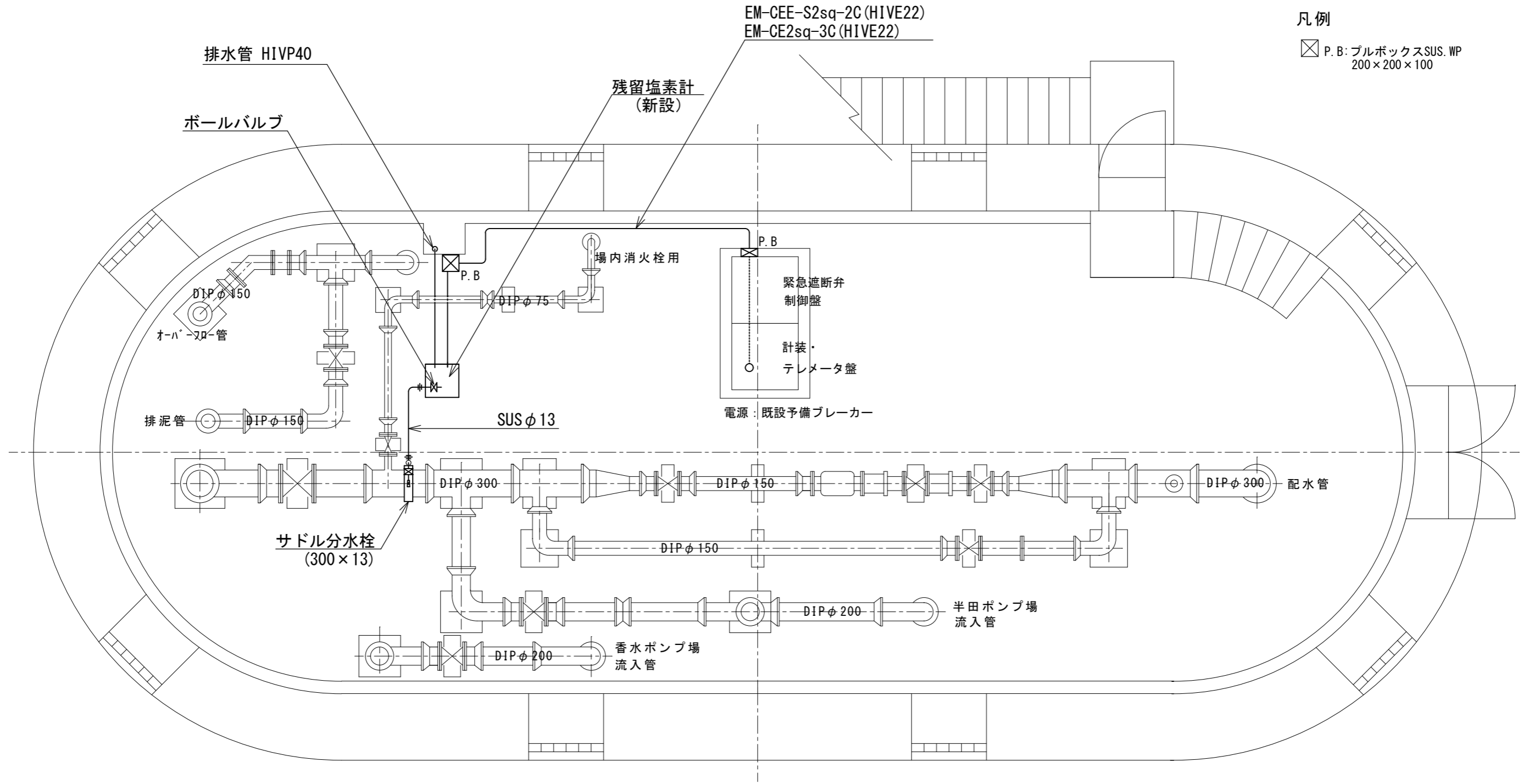
平面図
