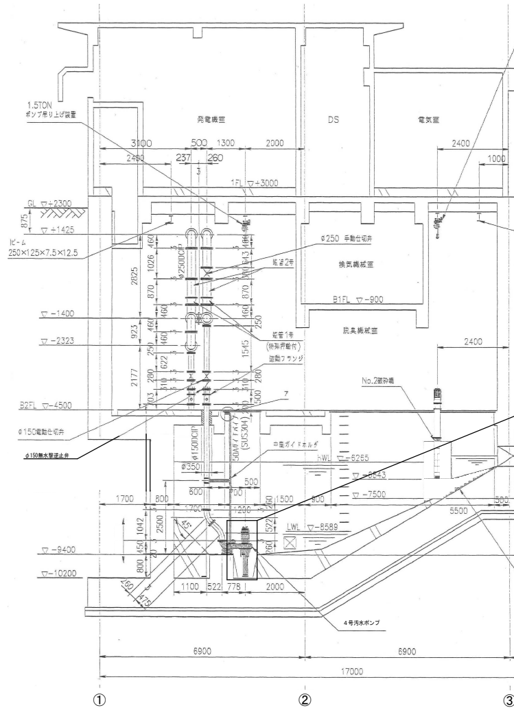
A-A断面図
