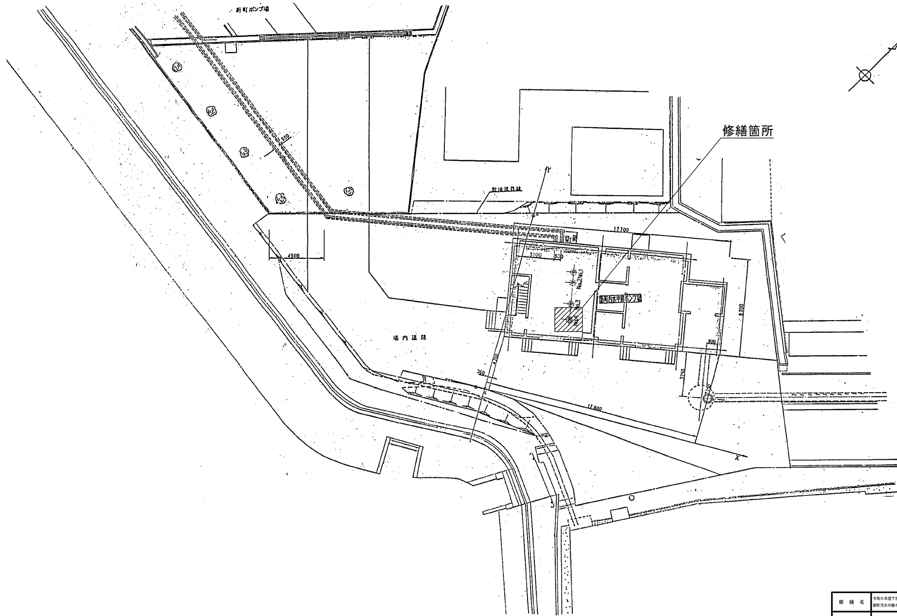
全体平面図
