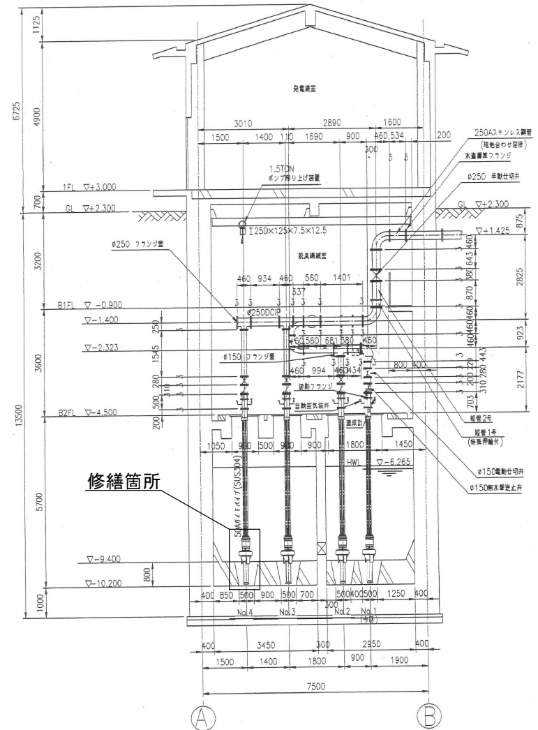
C-C断面図
