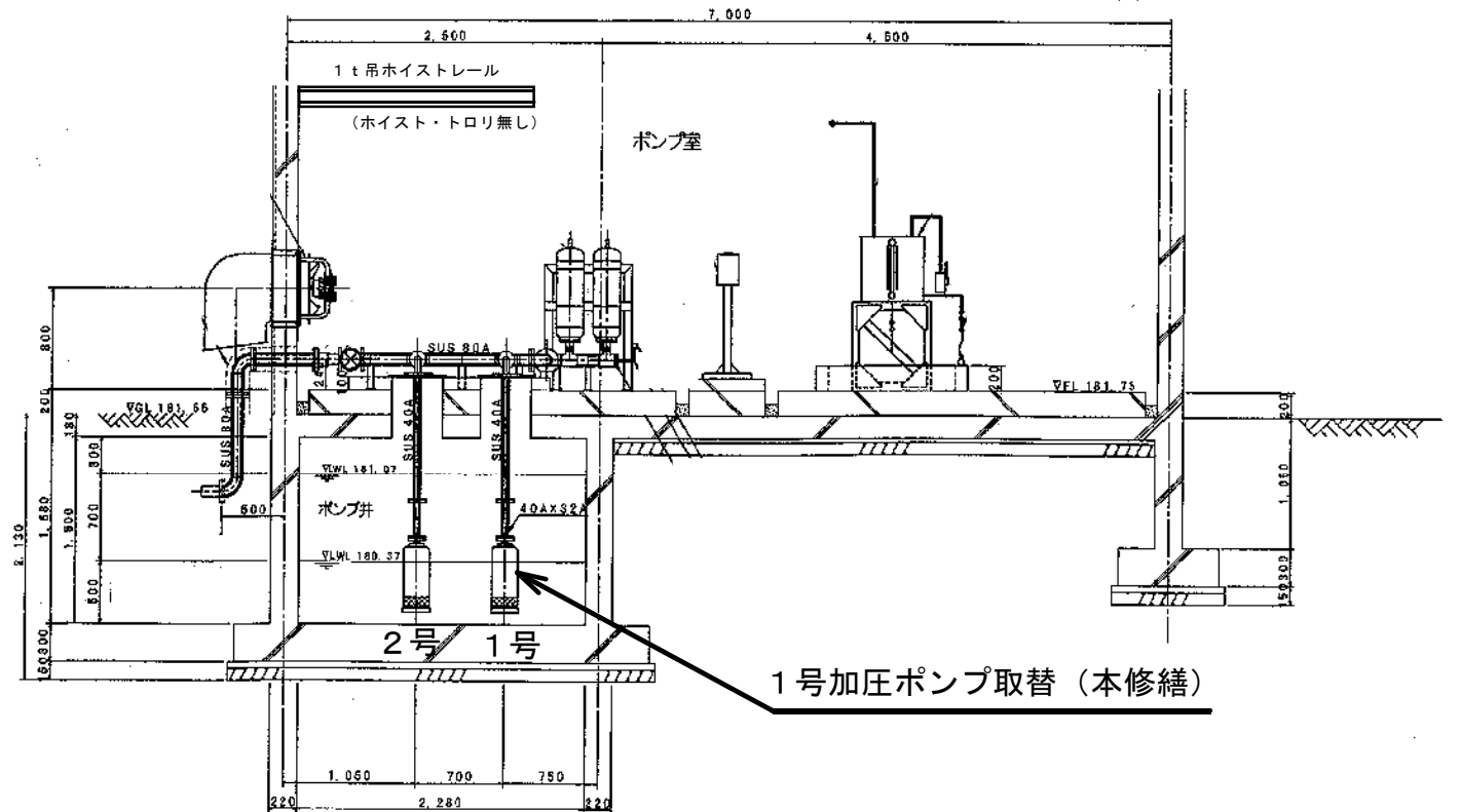
B-B断面図
