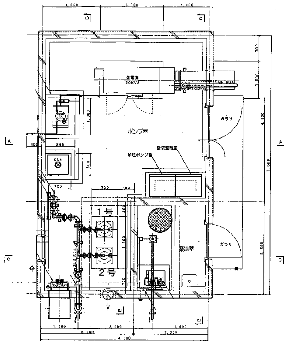
平面図
