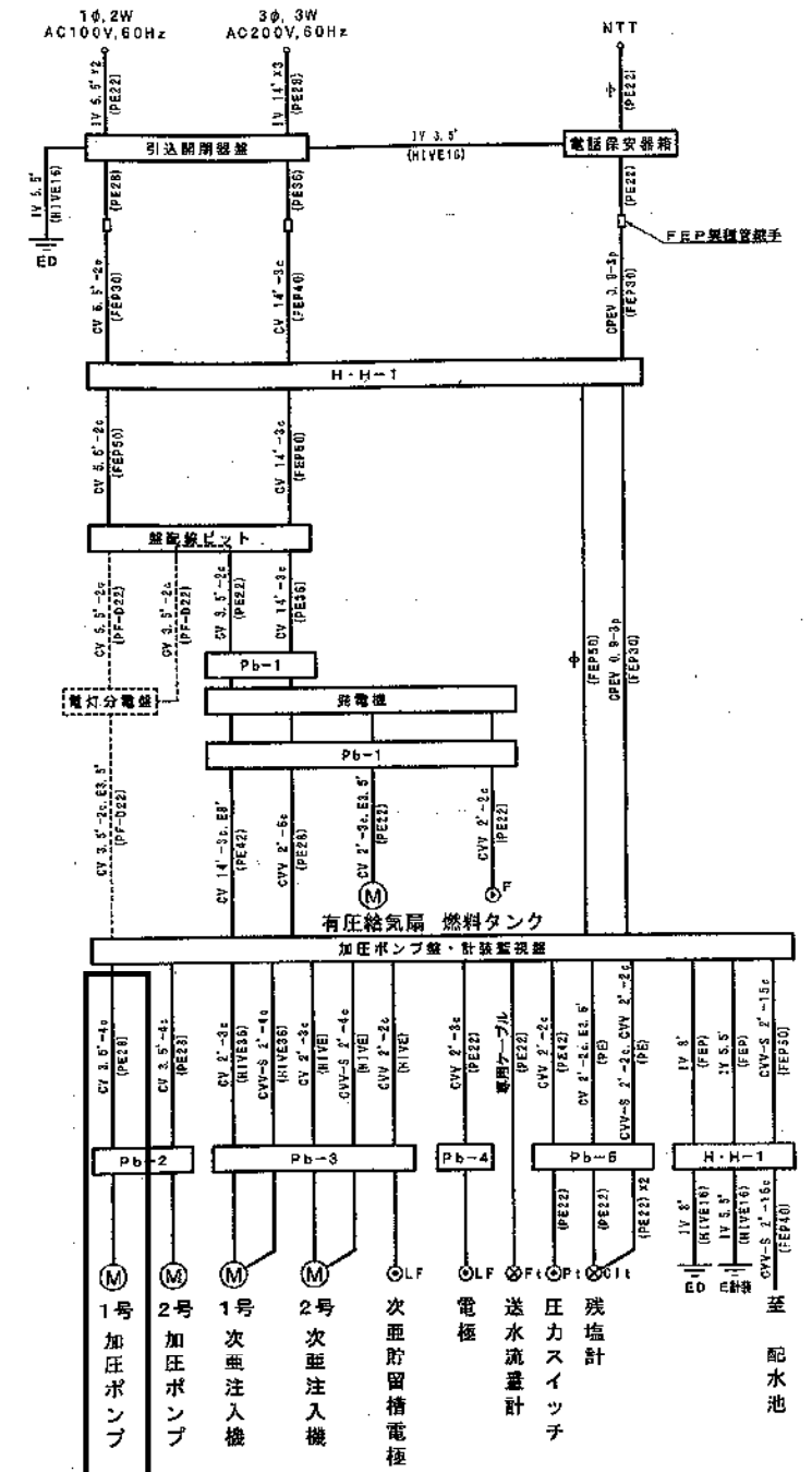
配線系統図
