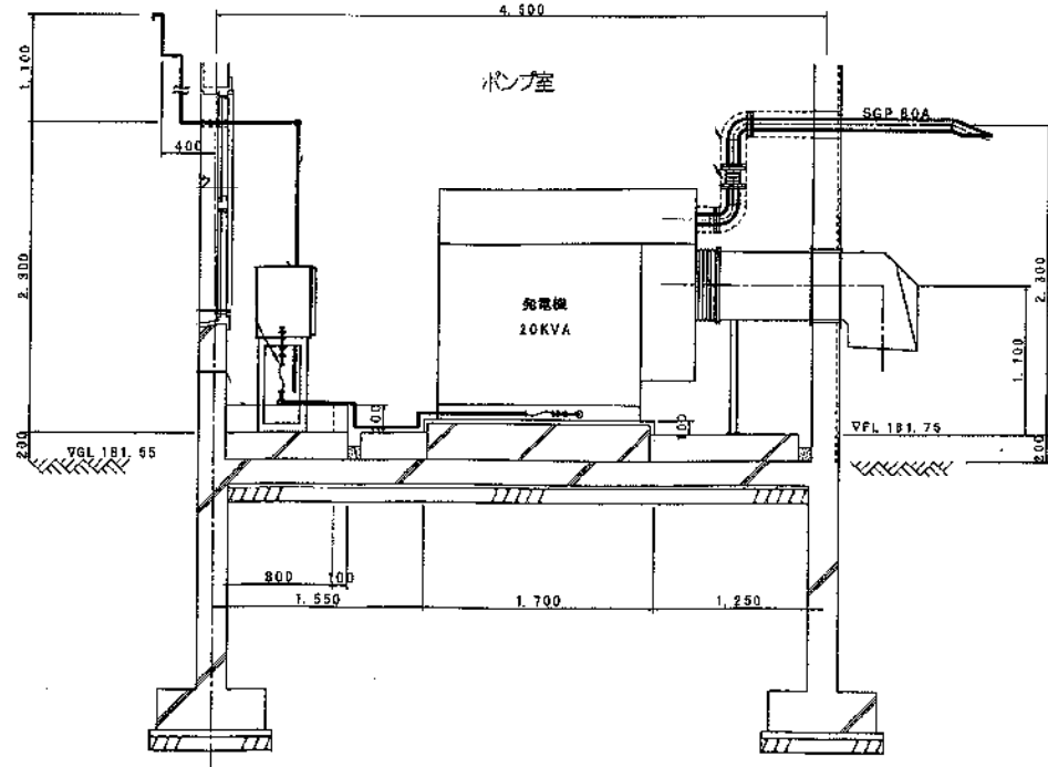
A-A断面図
