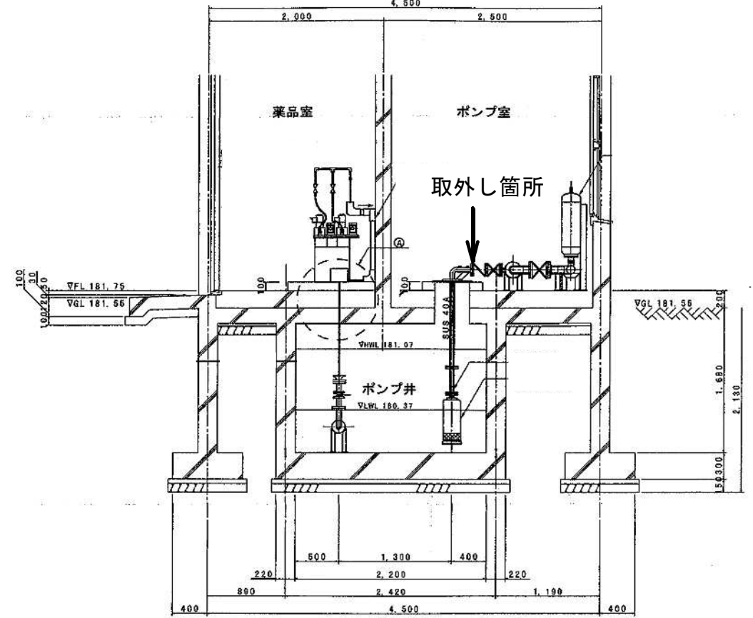
C-C断面図
