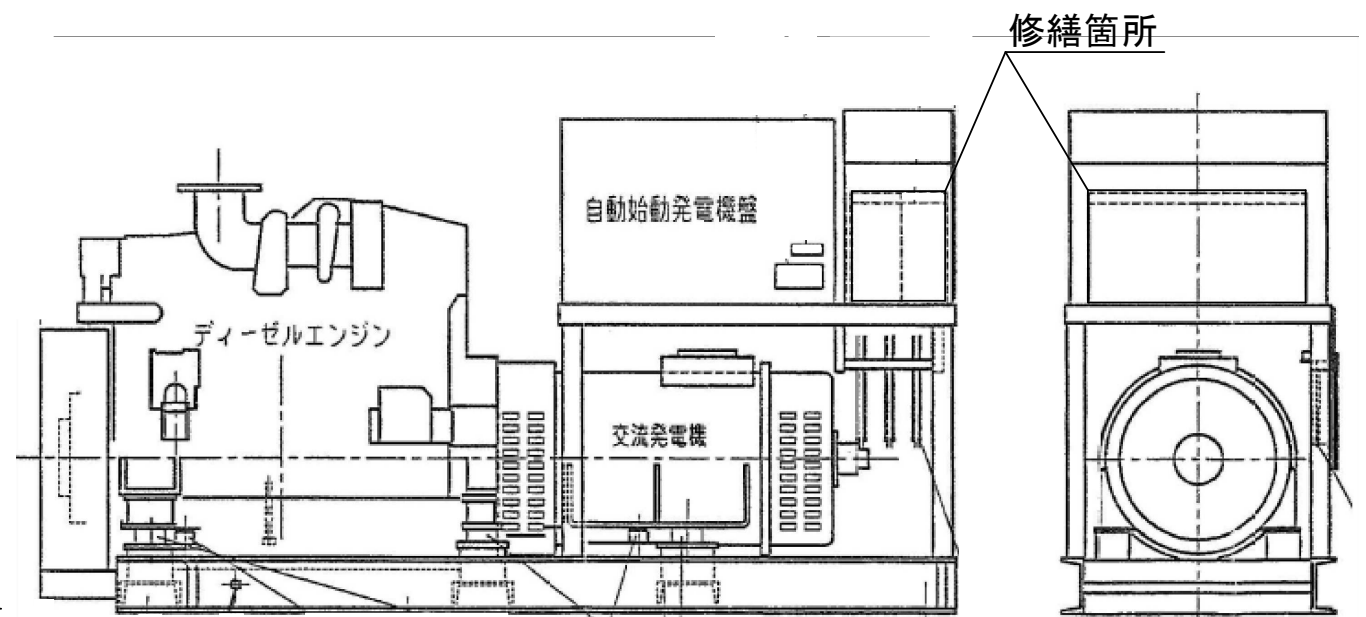
自家発電装置 外形図
