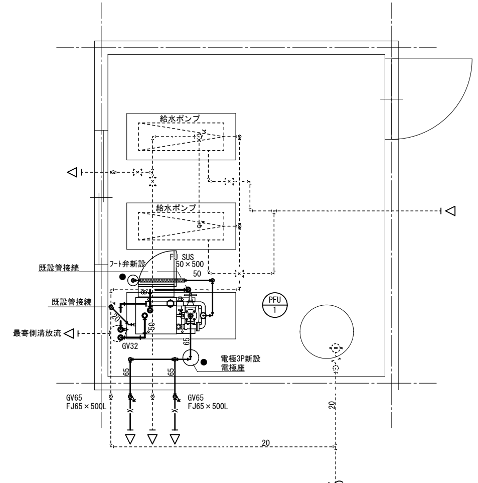
ポンプ室詳細図 S=1/30
