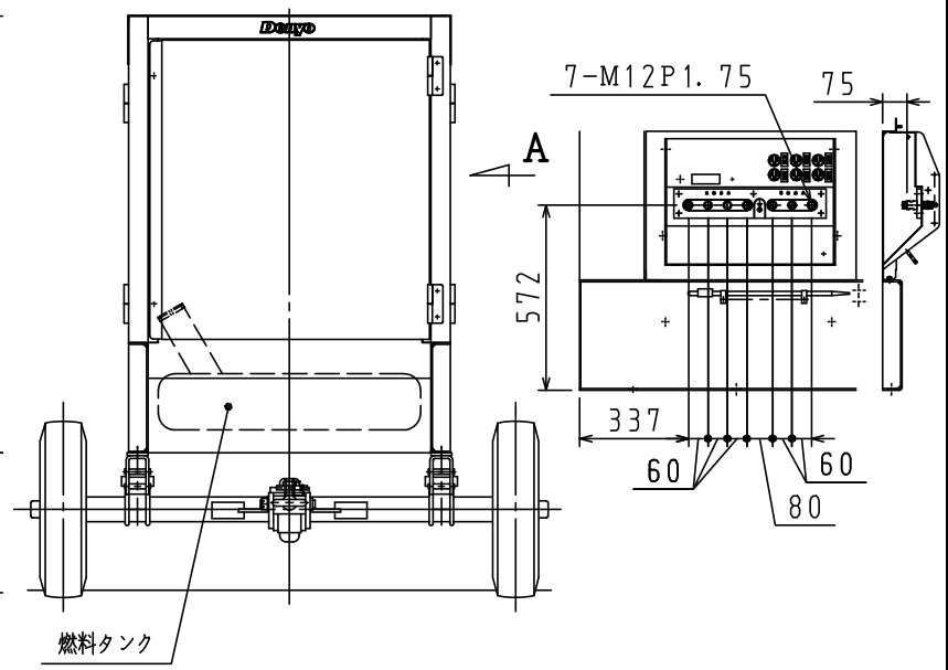
A 矢視図
