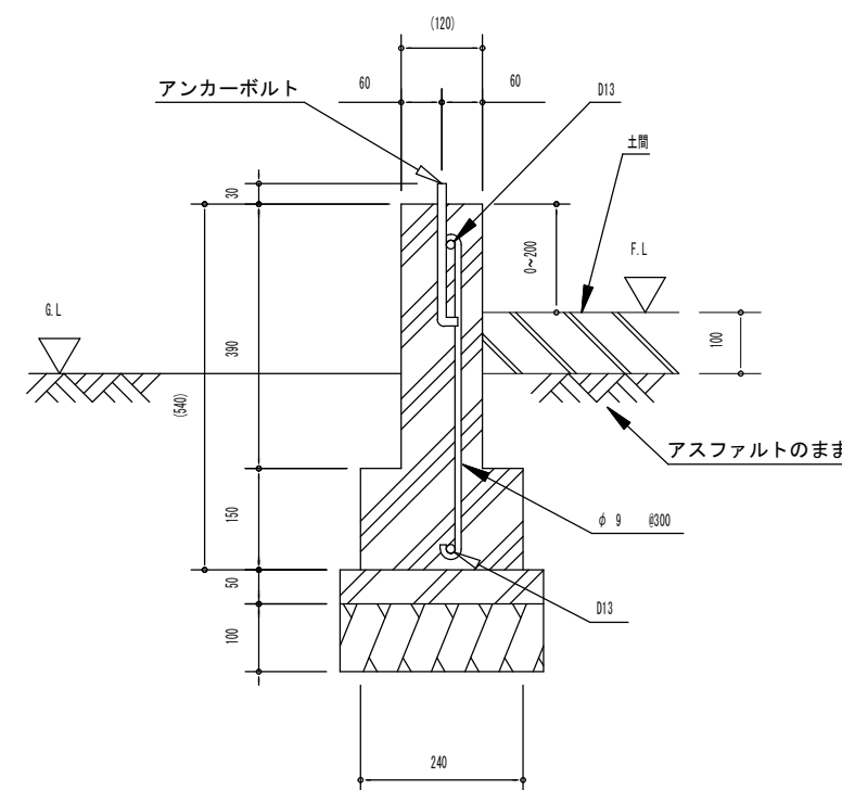
基礎詳細図 (1/20)
