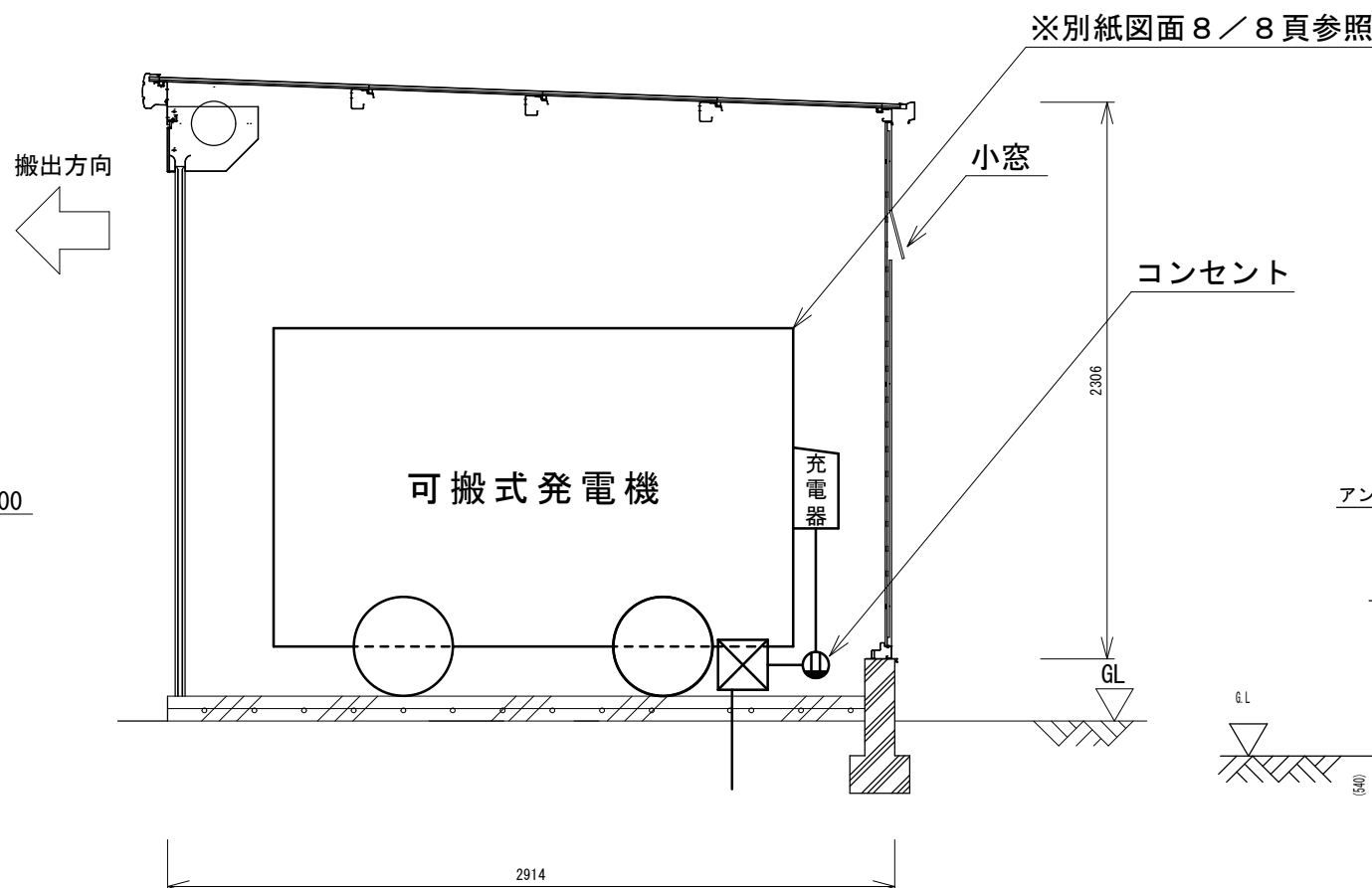
B - B 断面図
