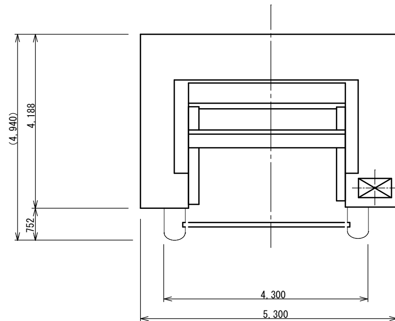
上面図
