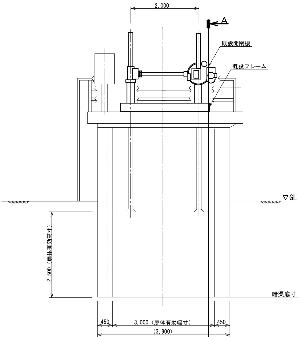
正面図
