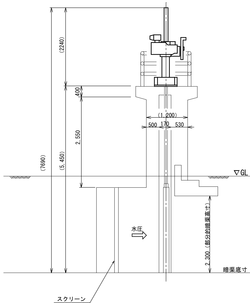
A-A断面図
