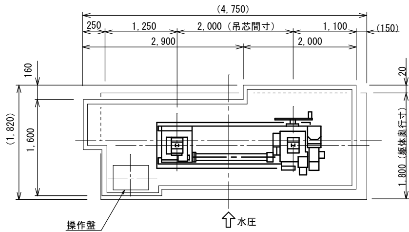
上面図
