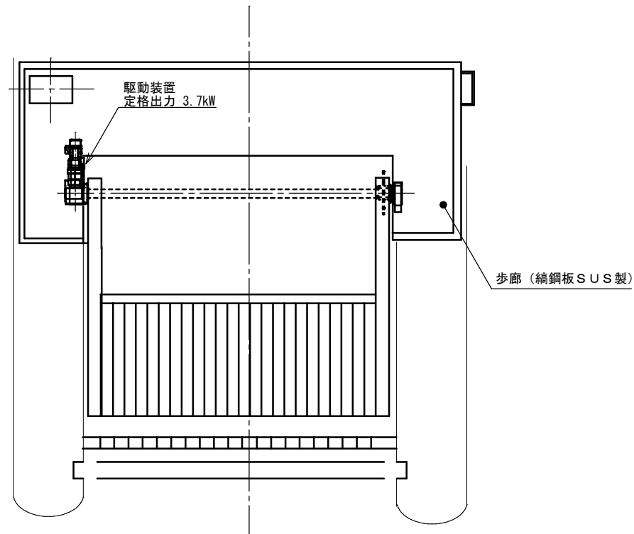
上面図
