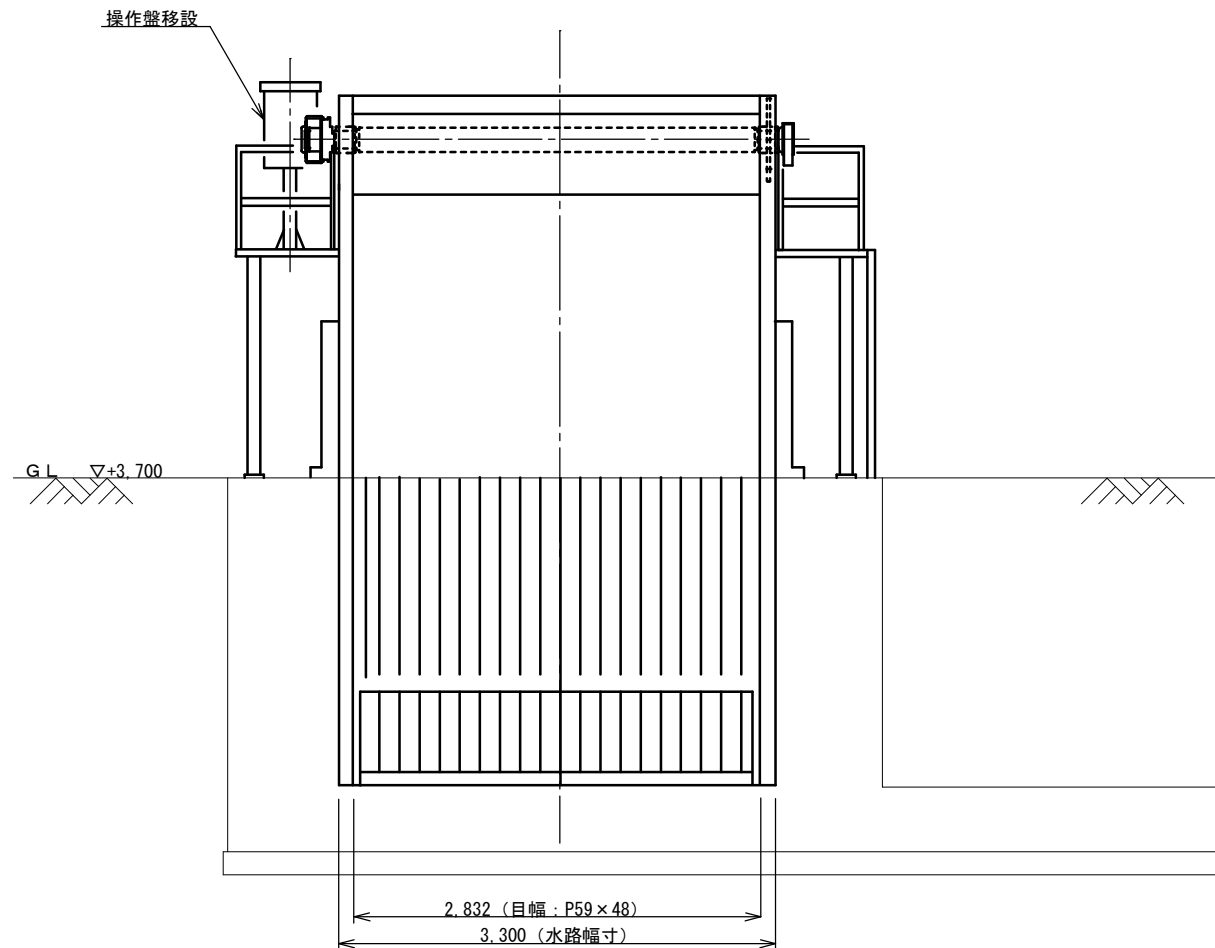
正面図
