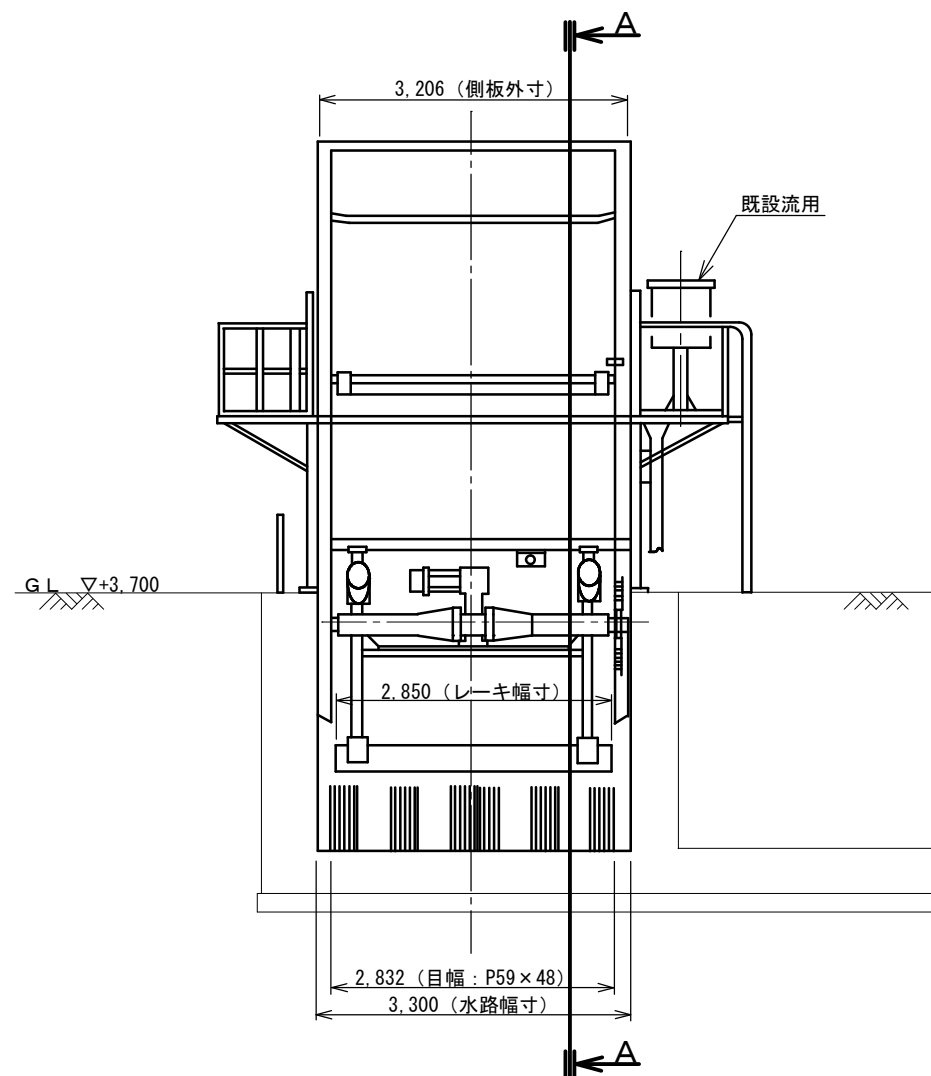
正面図
