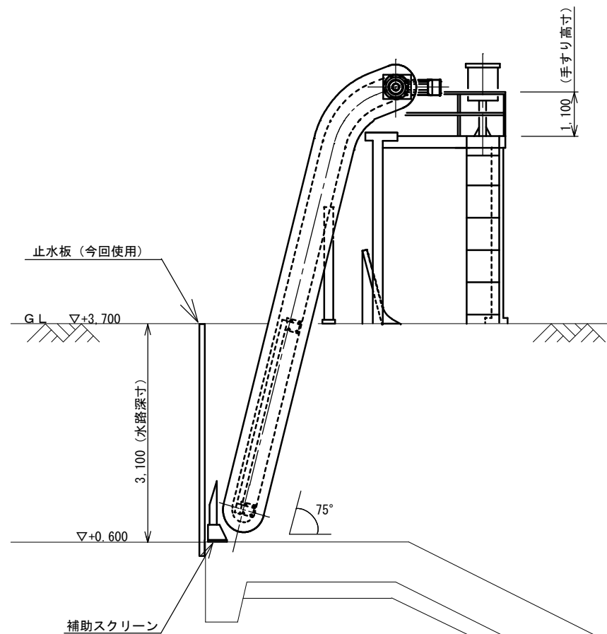
側面図
