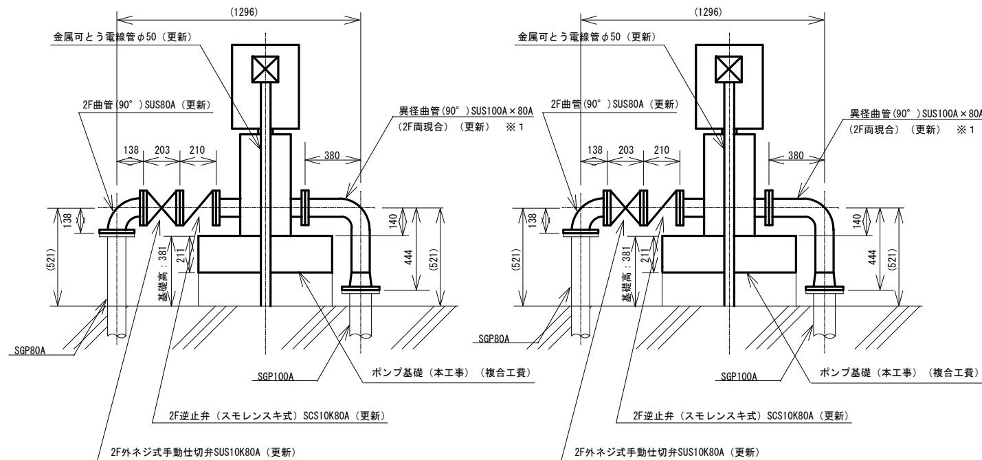
正面図（更新）
