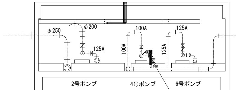
B-B断面図
