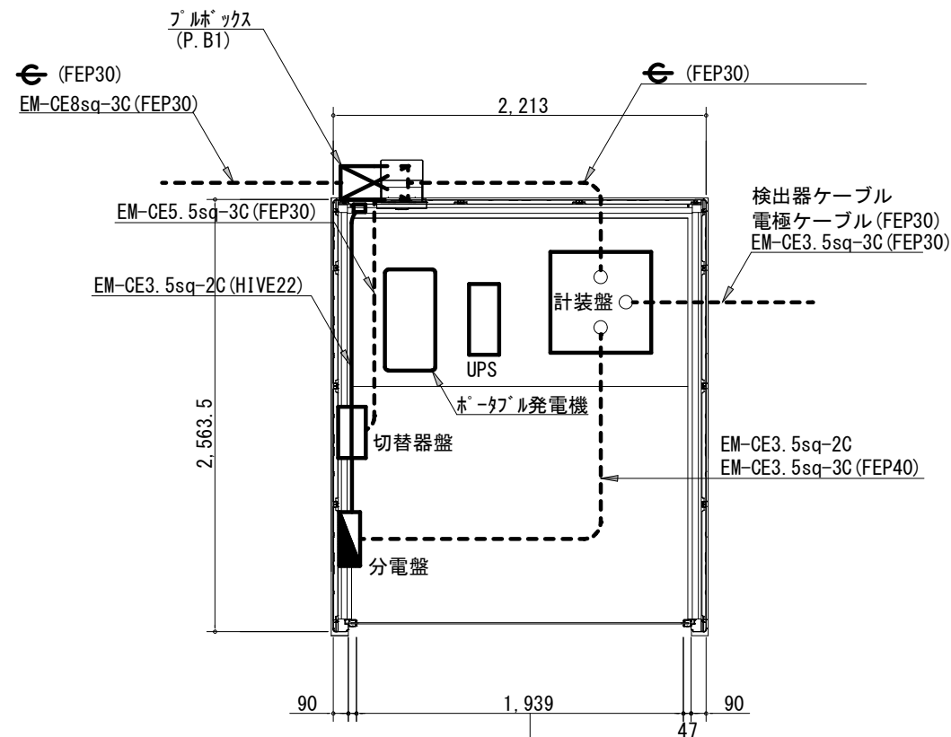
正面立面図 (1/40)
