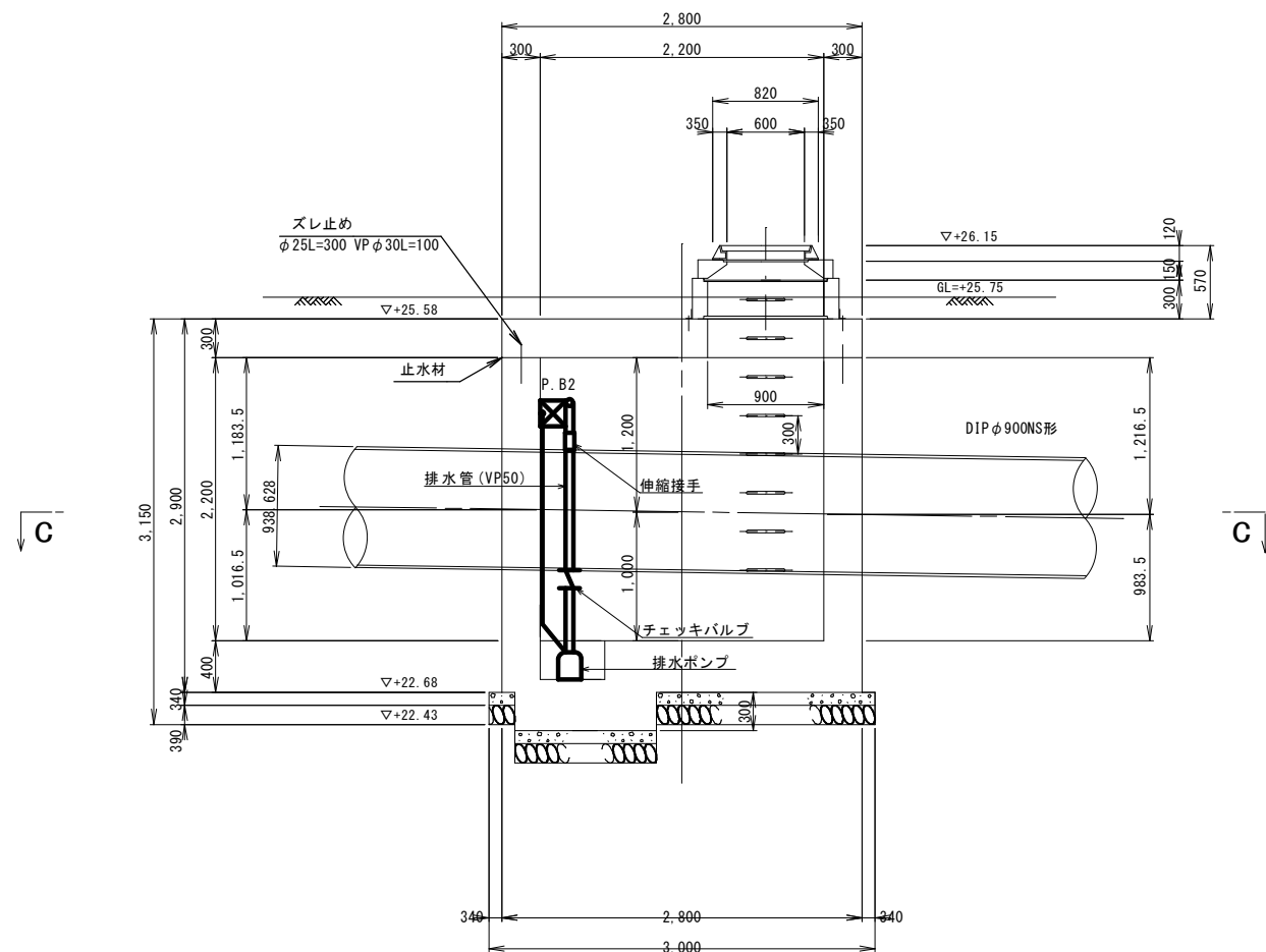
A-A断面図
