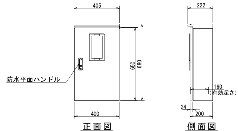
引込計器盤 S=1/20
