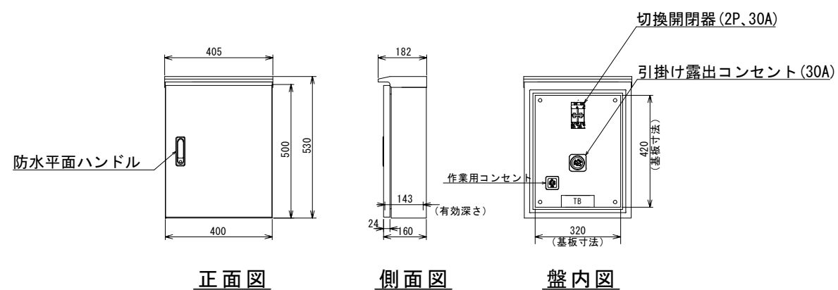
切換盤 S=1/20
