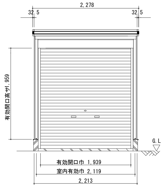
正面立面図 (1/40)
