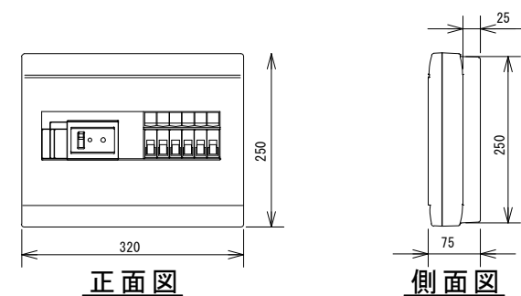
分電盤 S=1/10
