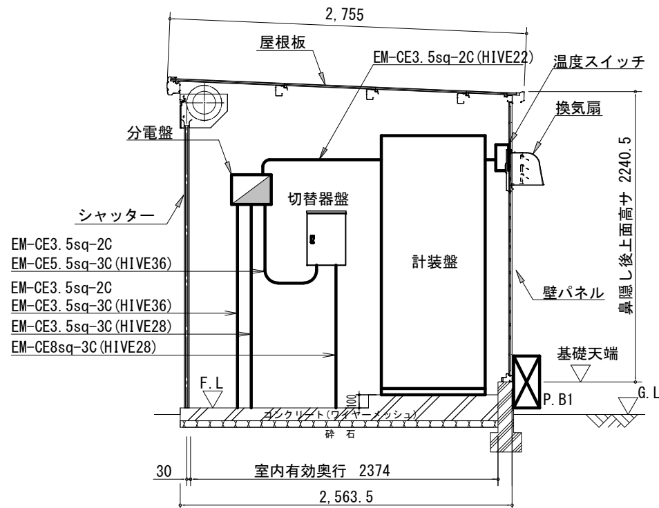
断面図 (1/40)
