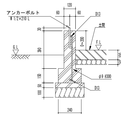
布基礎断面図例 (1/20)
