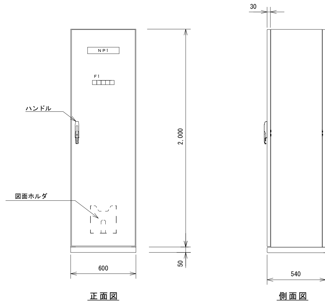
計装盤 S=1/20
