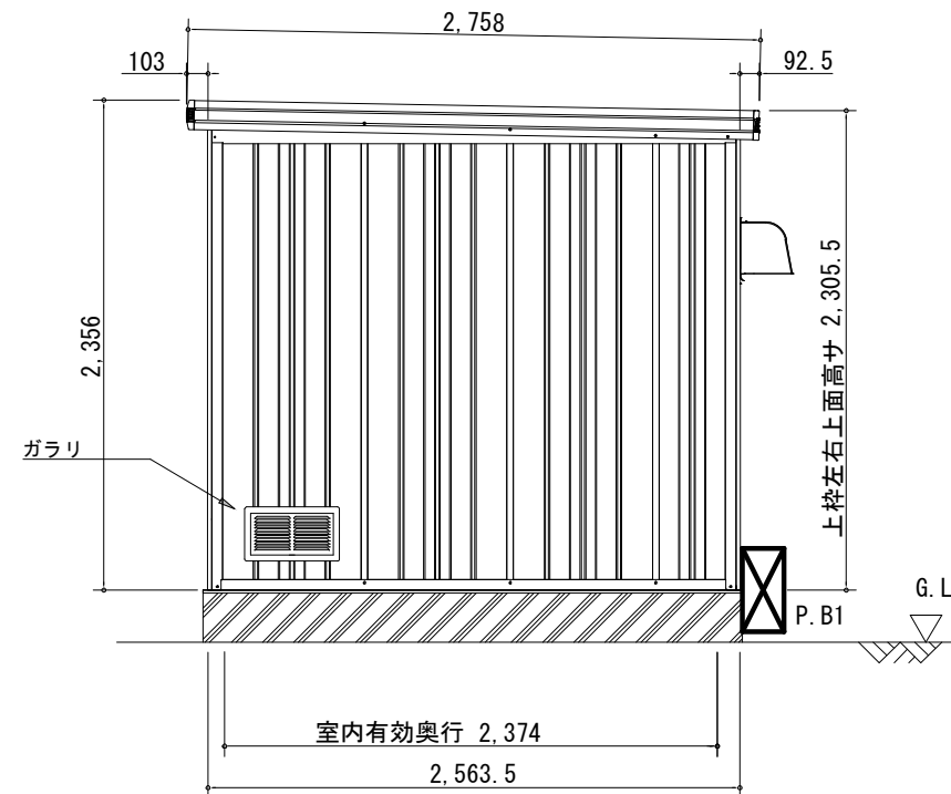
側面立面図 (1/40)
