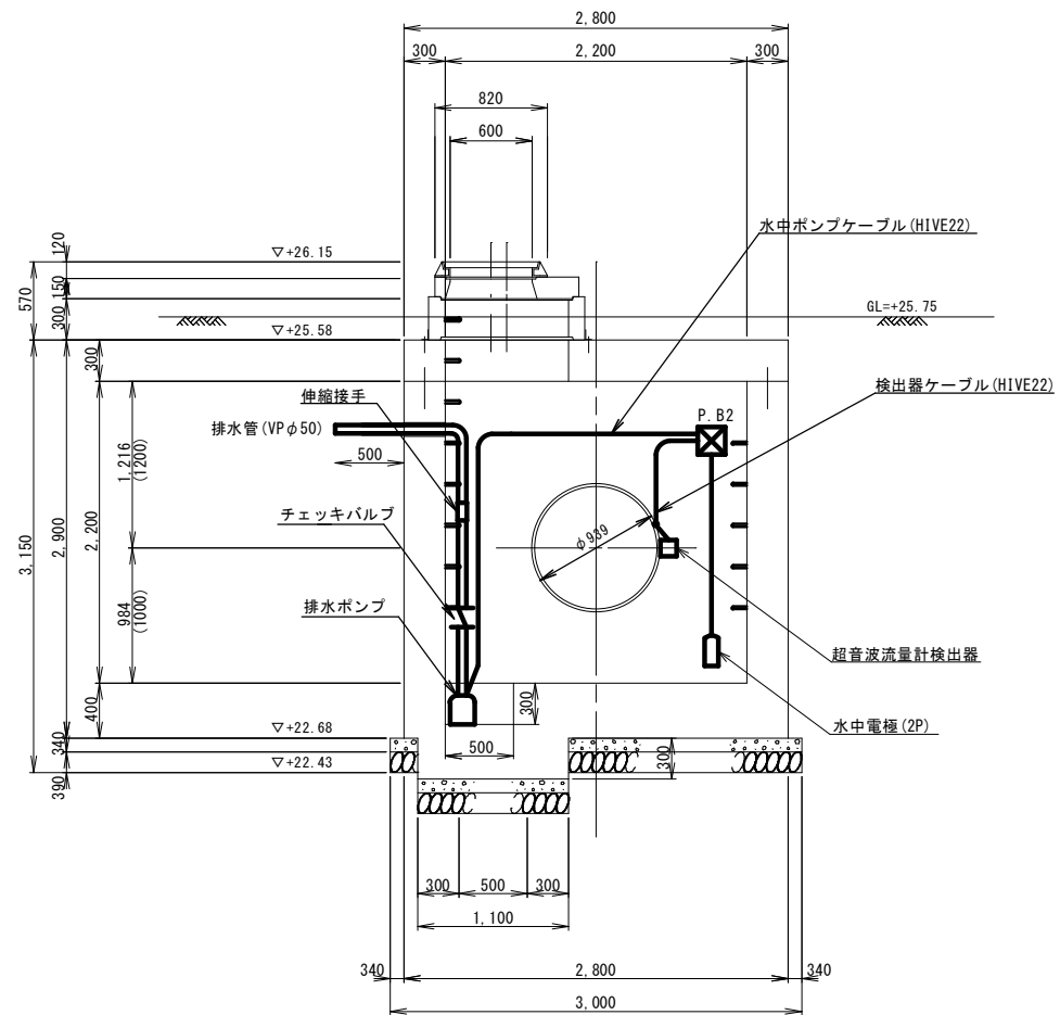
B-B断面図
