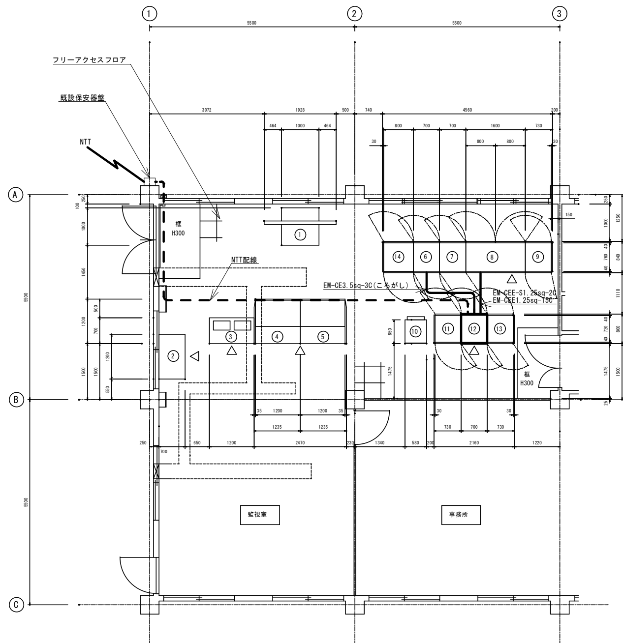
監視室 平面図 S=1/100
