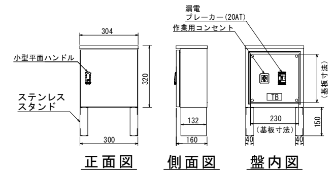
照明電源盤 S=1/20
