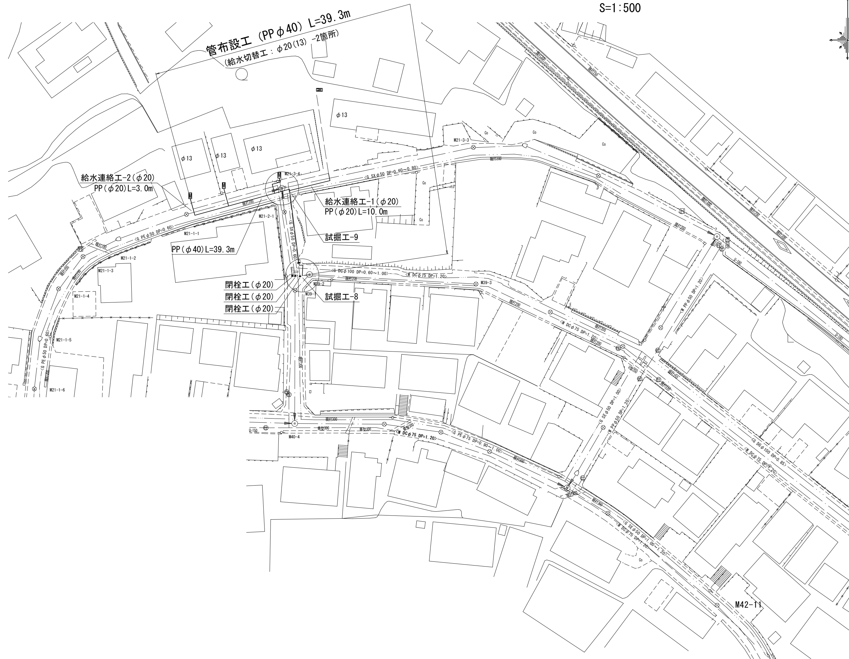
平面図
