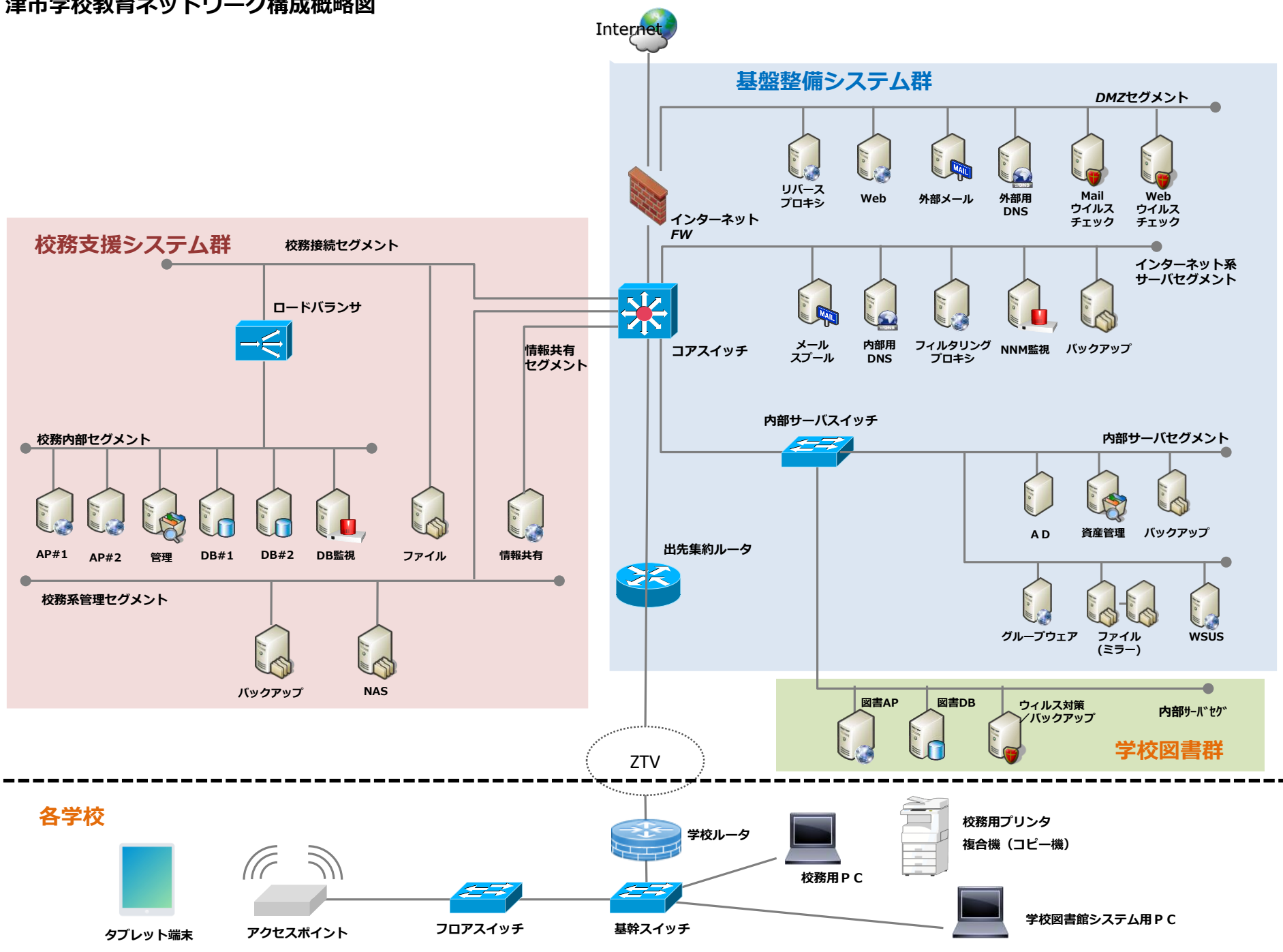
津市学校教育ネットワーク構成概略図
