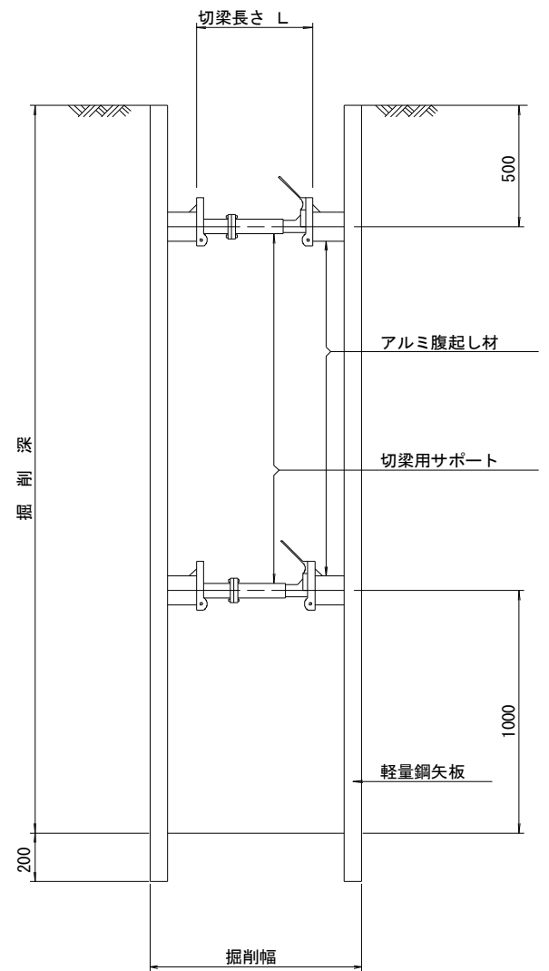
断面図 S=1/20
