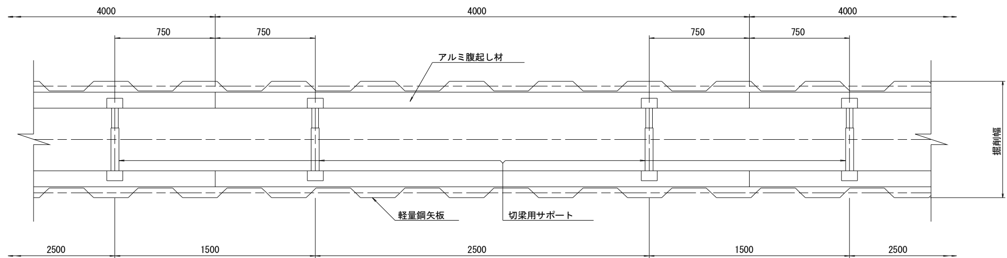
平面図 S=1/20
