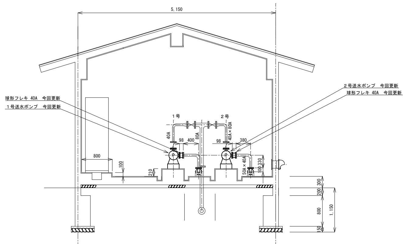
A-A断面図
