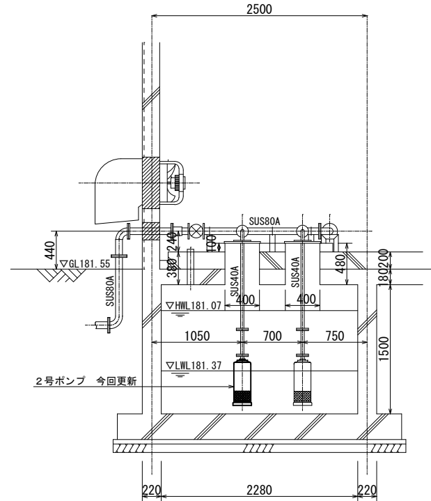
B - B 断面図
