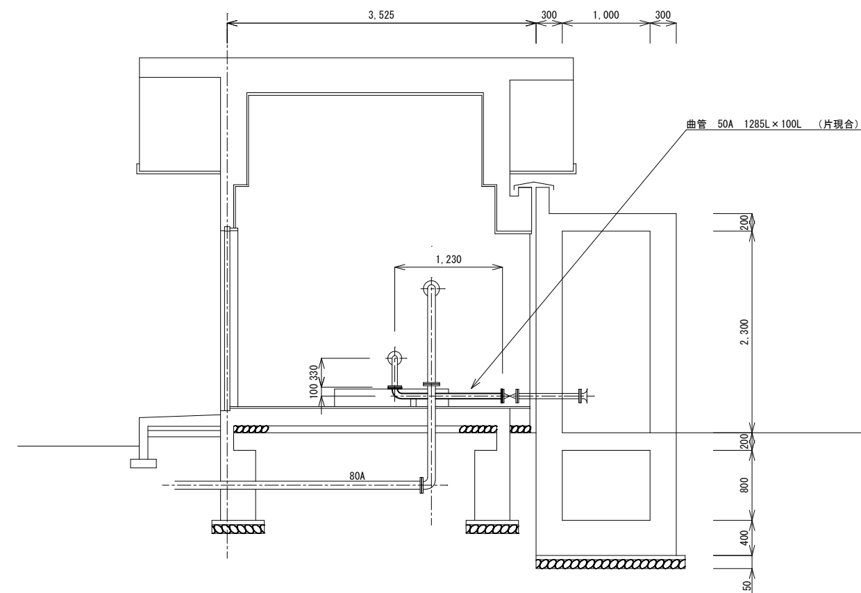
矢視B
