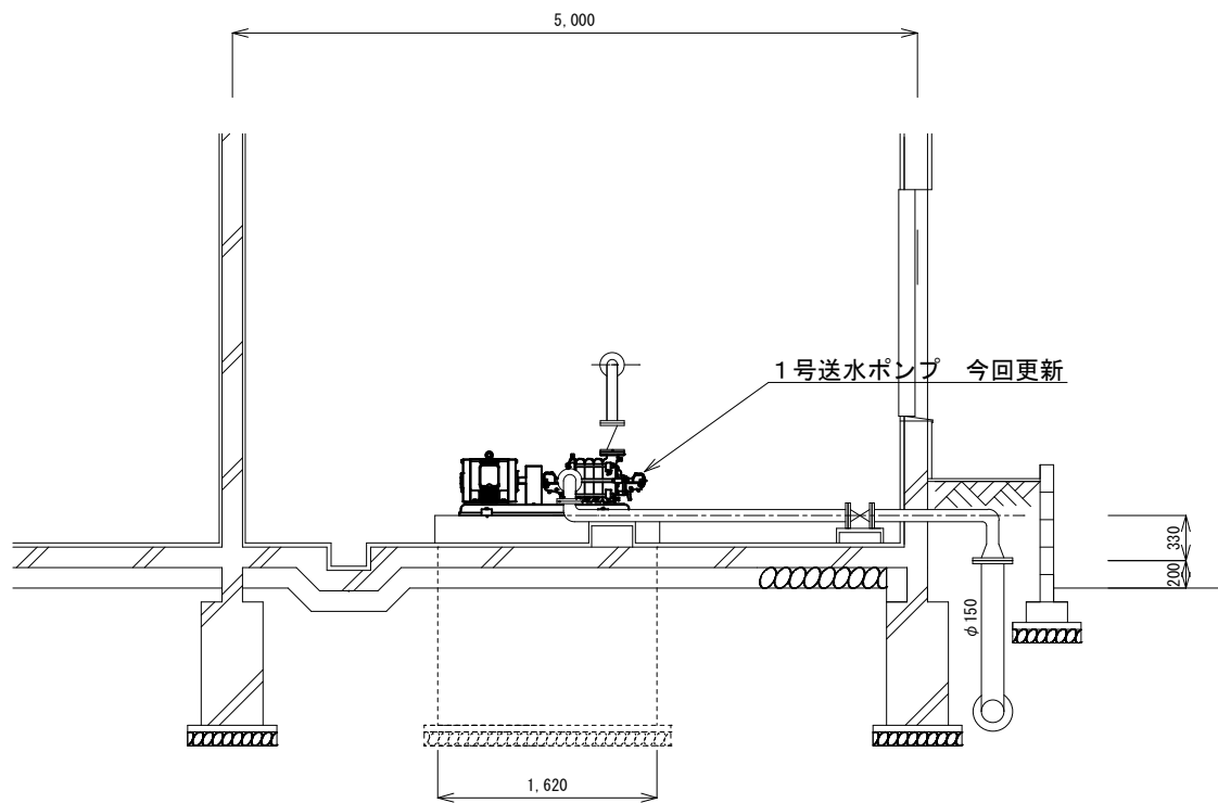
A-A断面図
