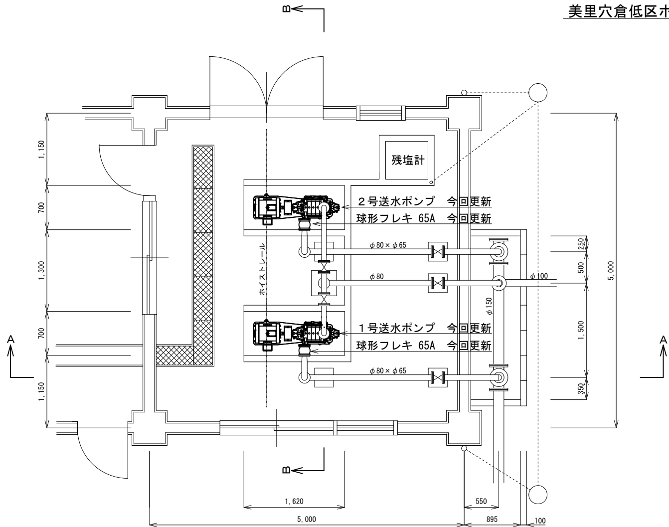
平面図
