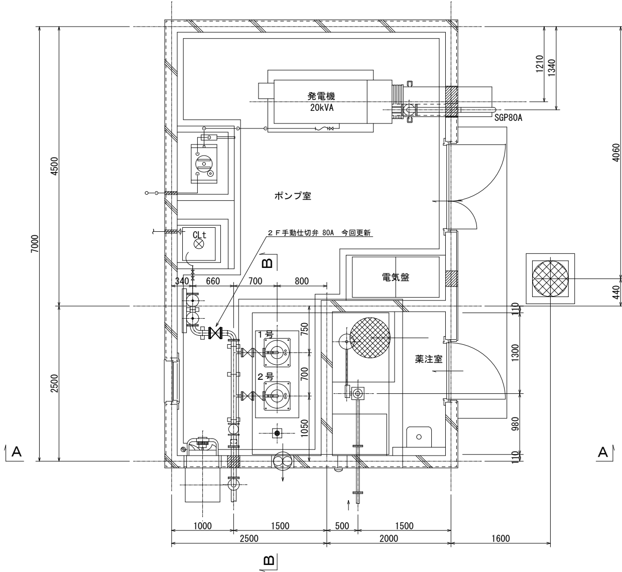
平面図
