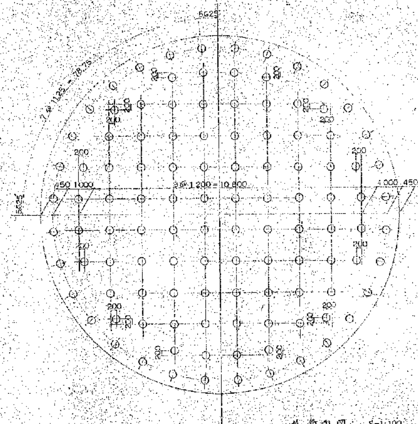
杭頭詳細図 S=1:100 (第1次設計) 1/1
