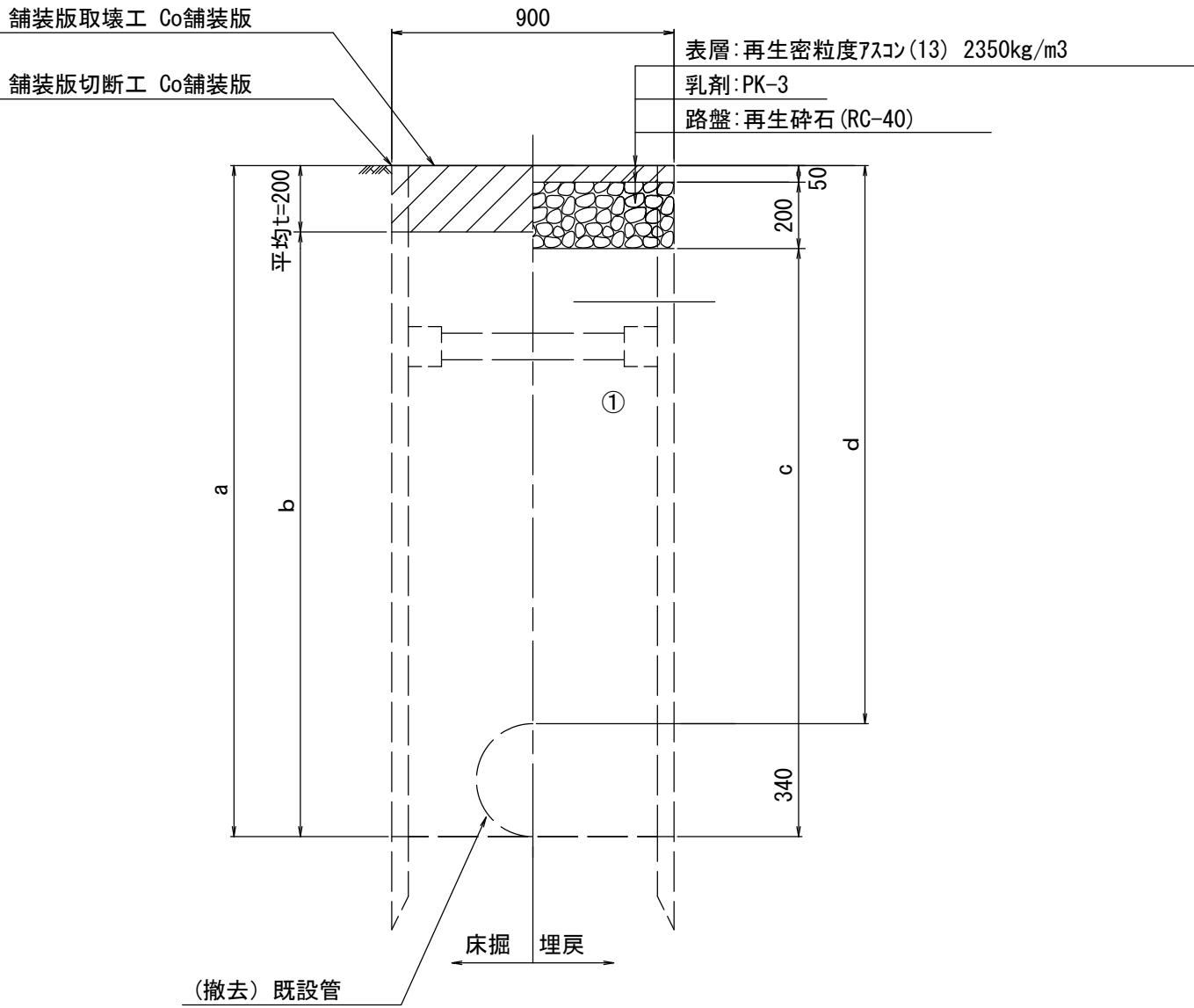
既設管撤去
