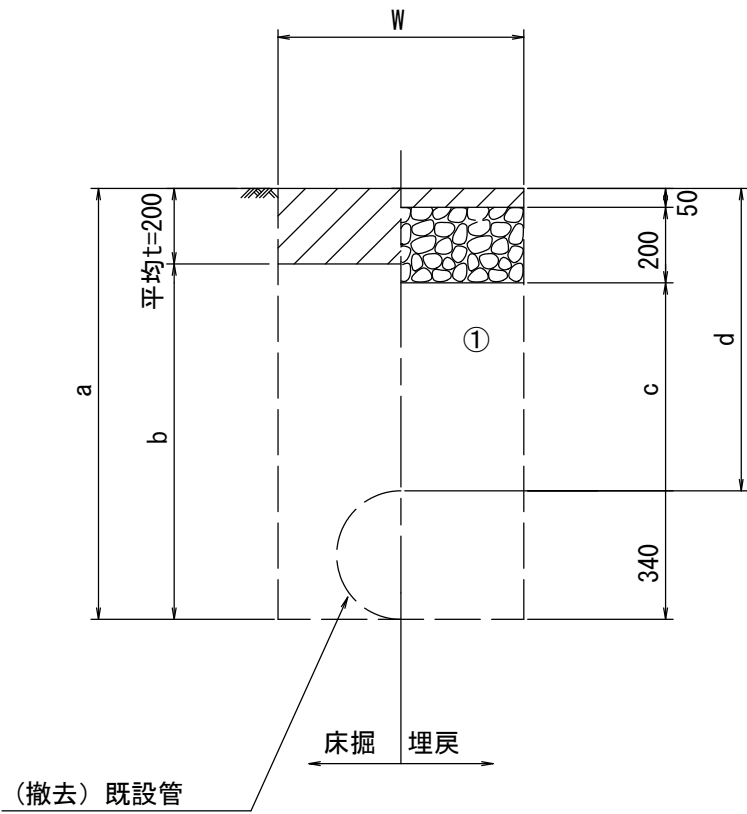
既設管撤去
