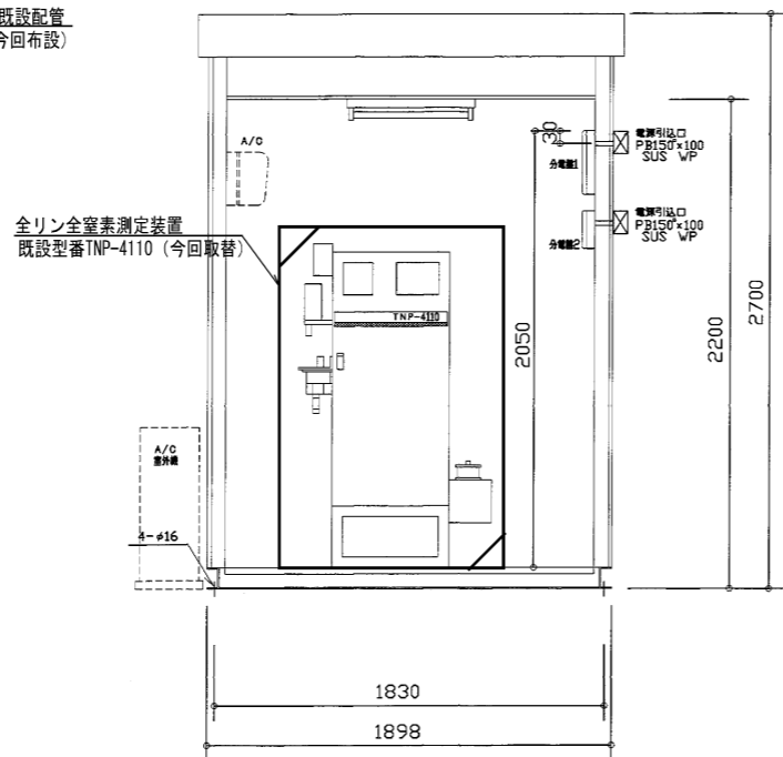
A-A 矢視図
