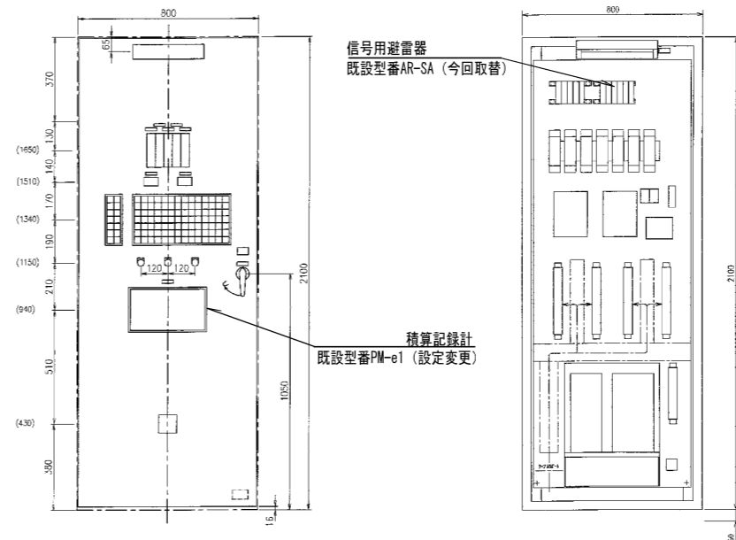
監視計装盤面配置図 (前面)
