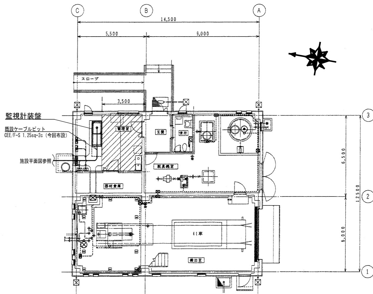
管理棟平面詳細図
