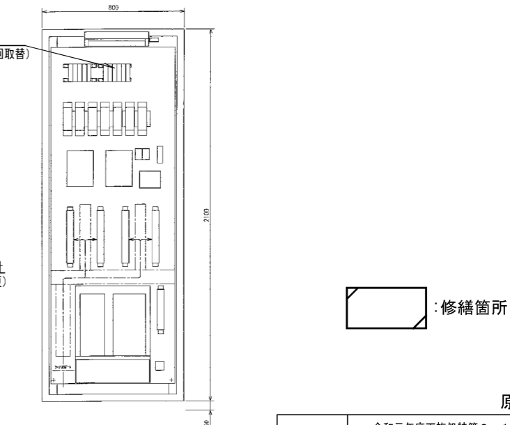
監視計装盤器具配置図 (前面)
