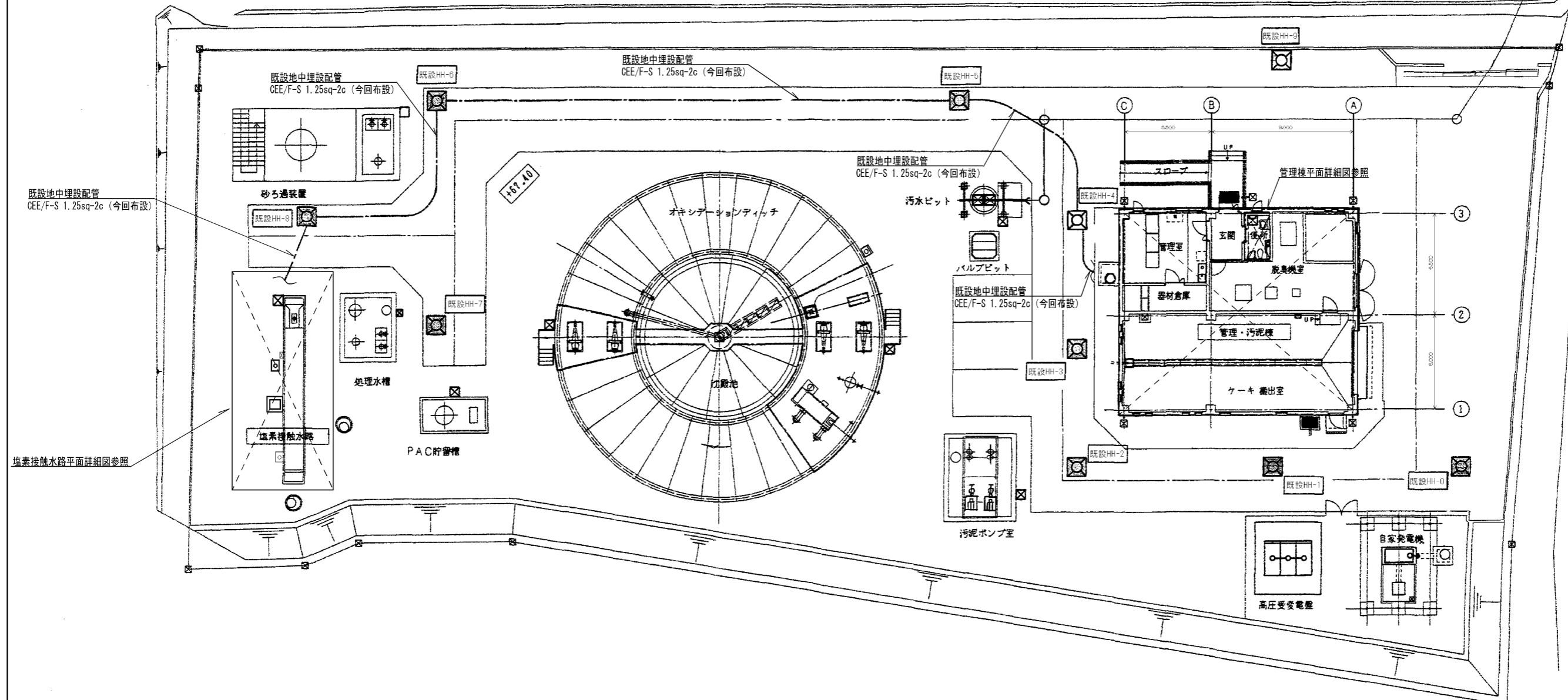
施設平面図
