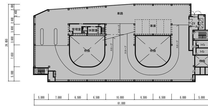
2階平面図
