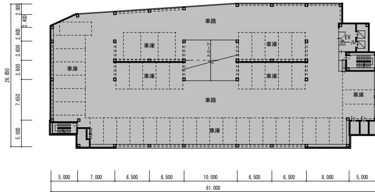
6～9階平面図
