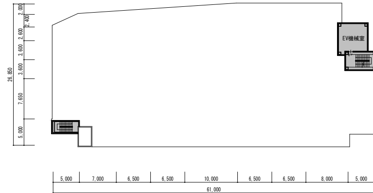
PH2階平面図
