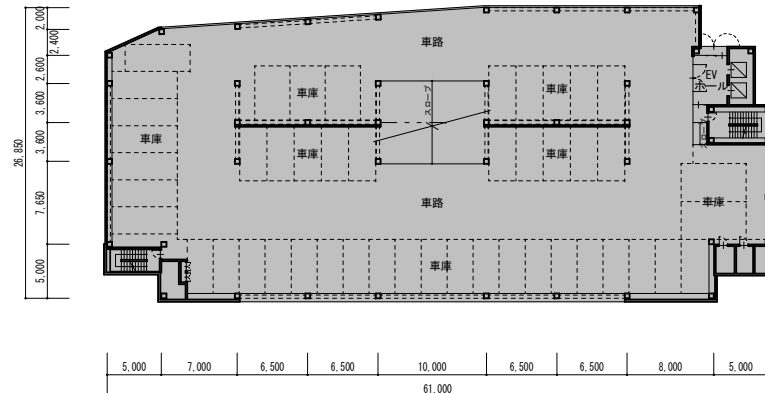
3~5階平面図
