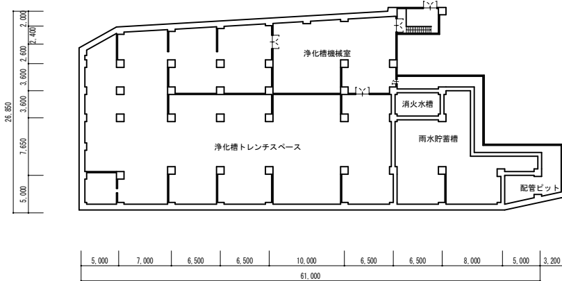
地階平面図
