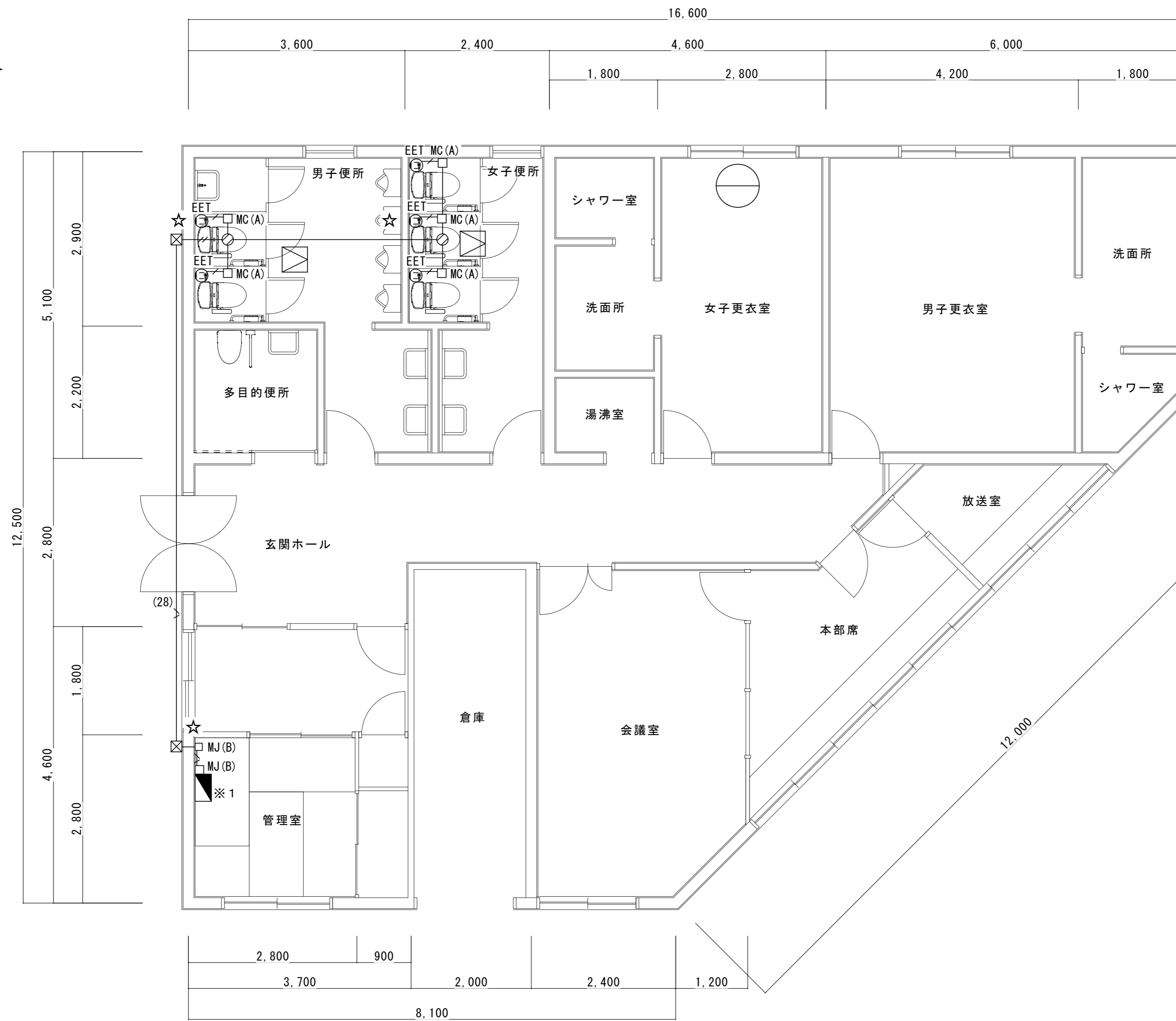
平面図 S=1/50
