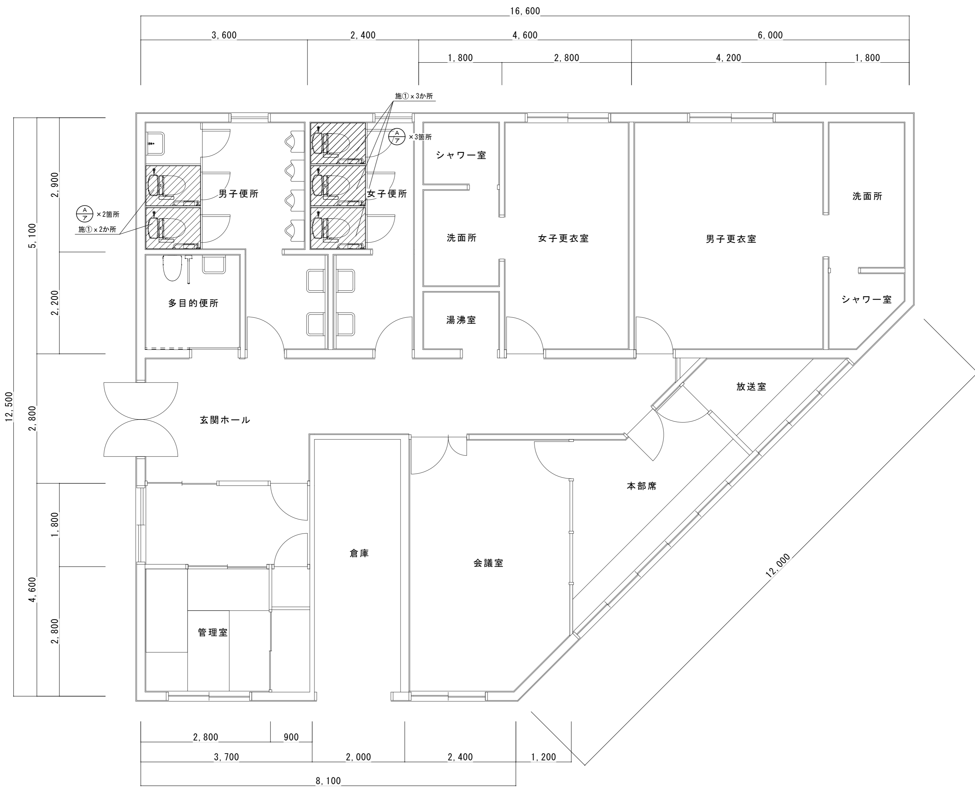
平面図 S=1/50
