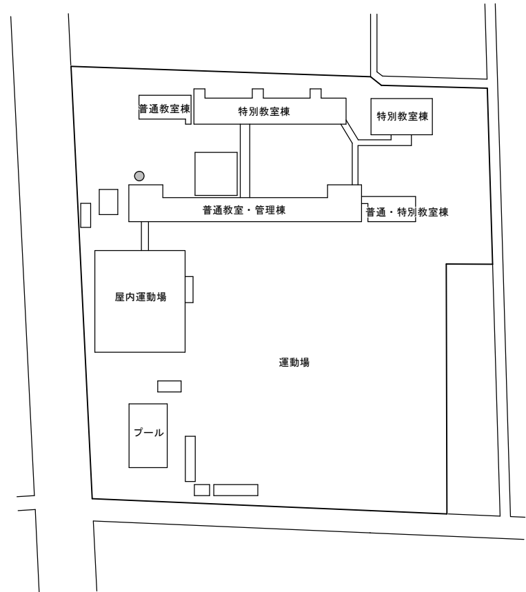
配置図
