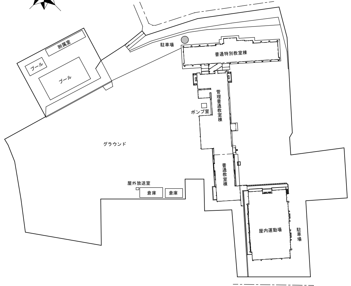
配置図
