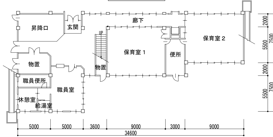
2階平面図
