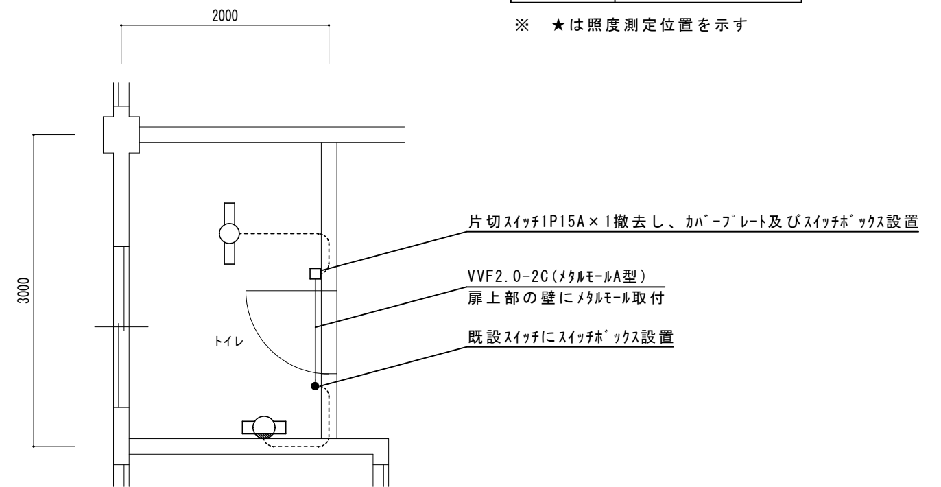
平面詳細図 1/50
