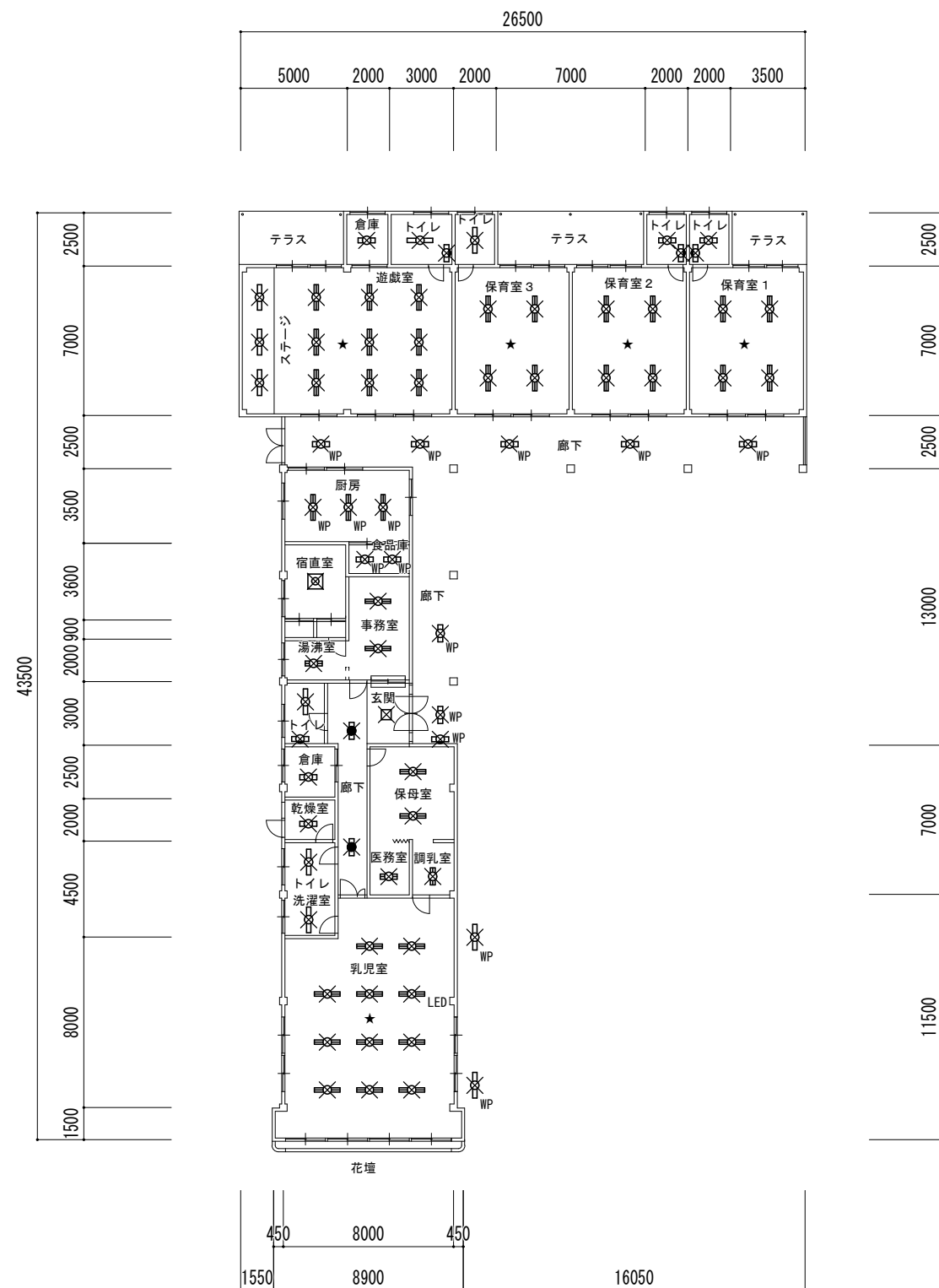
平面図 1/300
