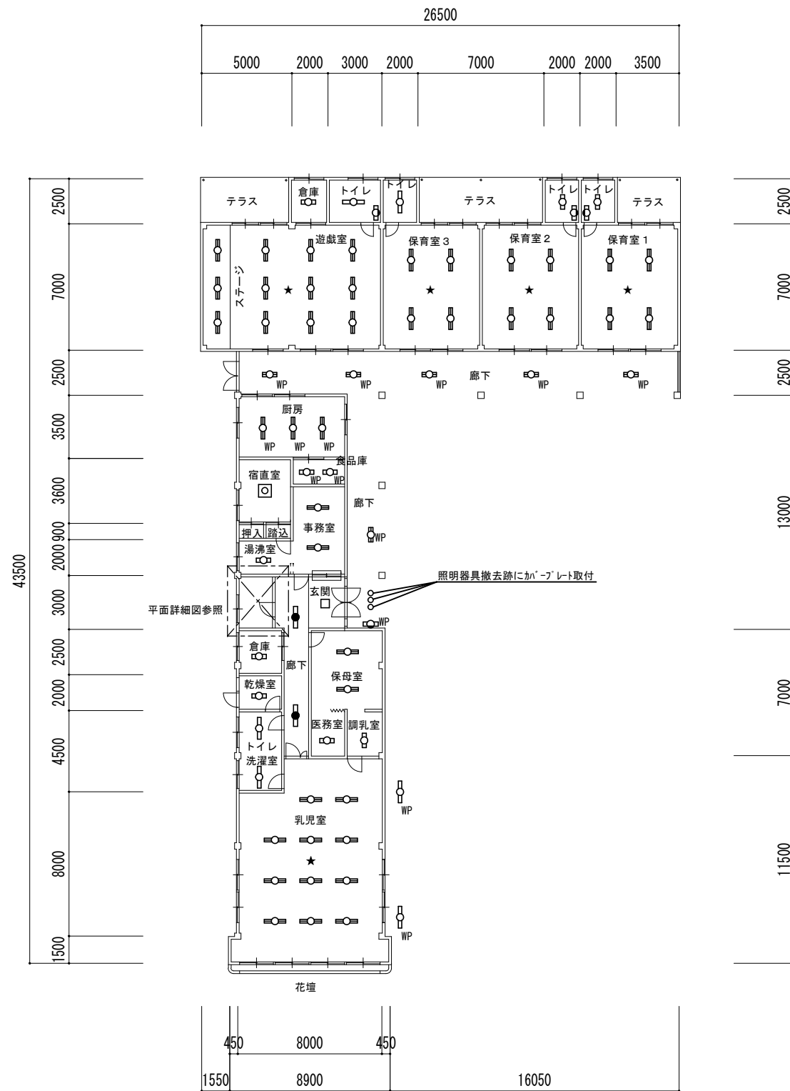
平面図 1/300
