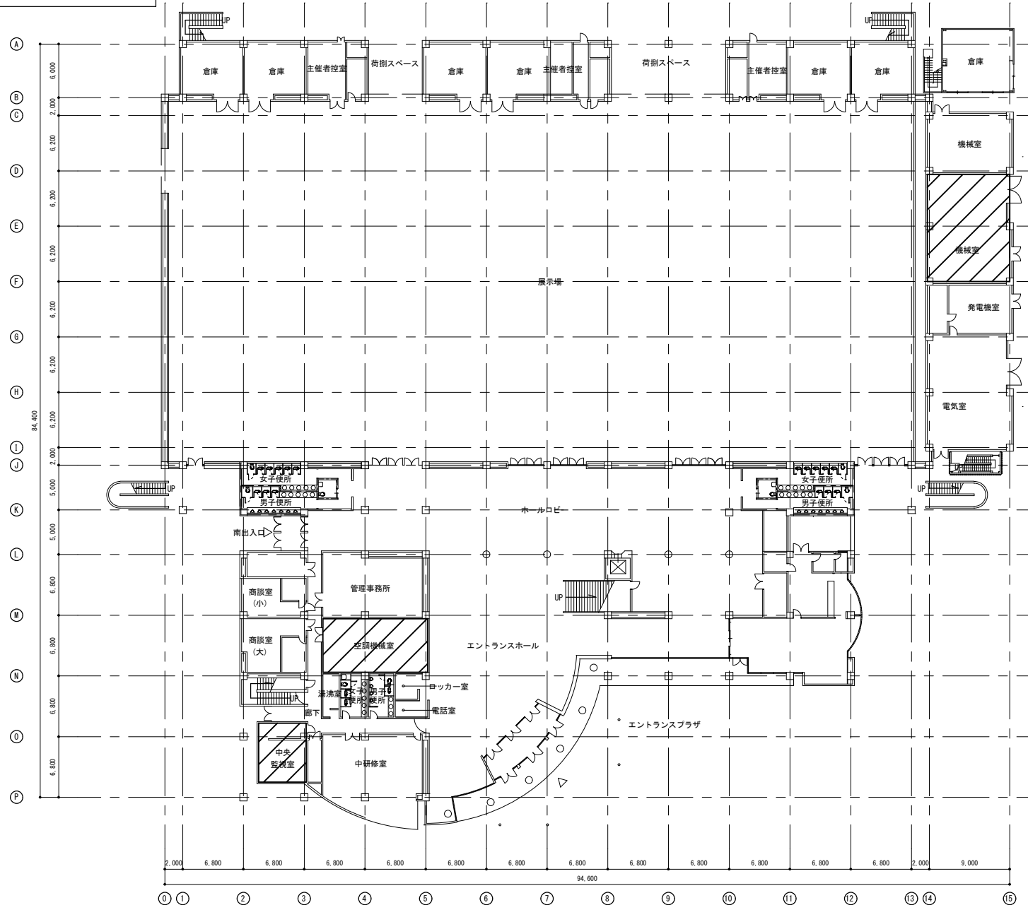
1階平面図
