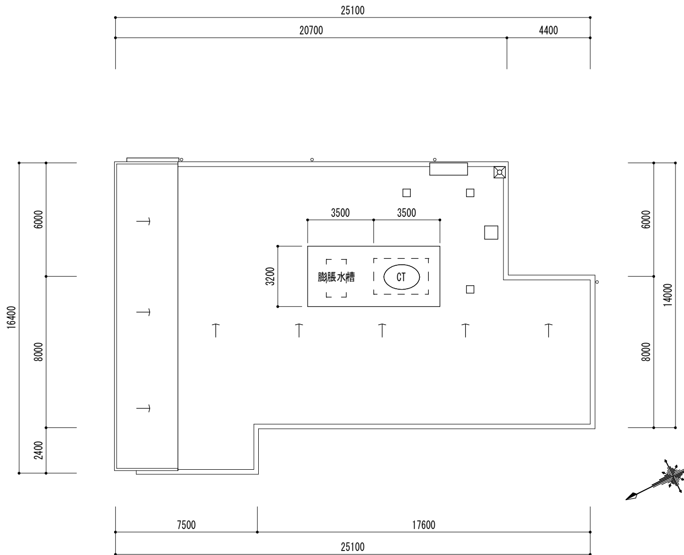
R階平面図
