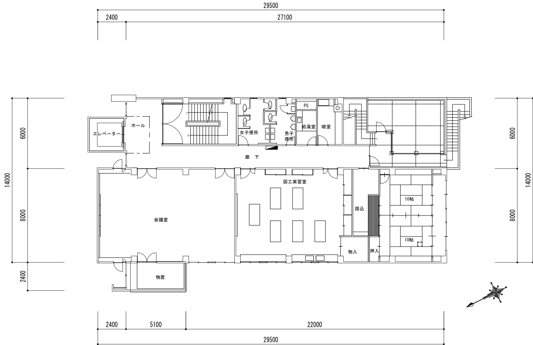
2階平面図
