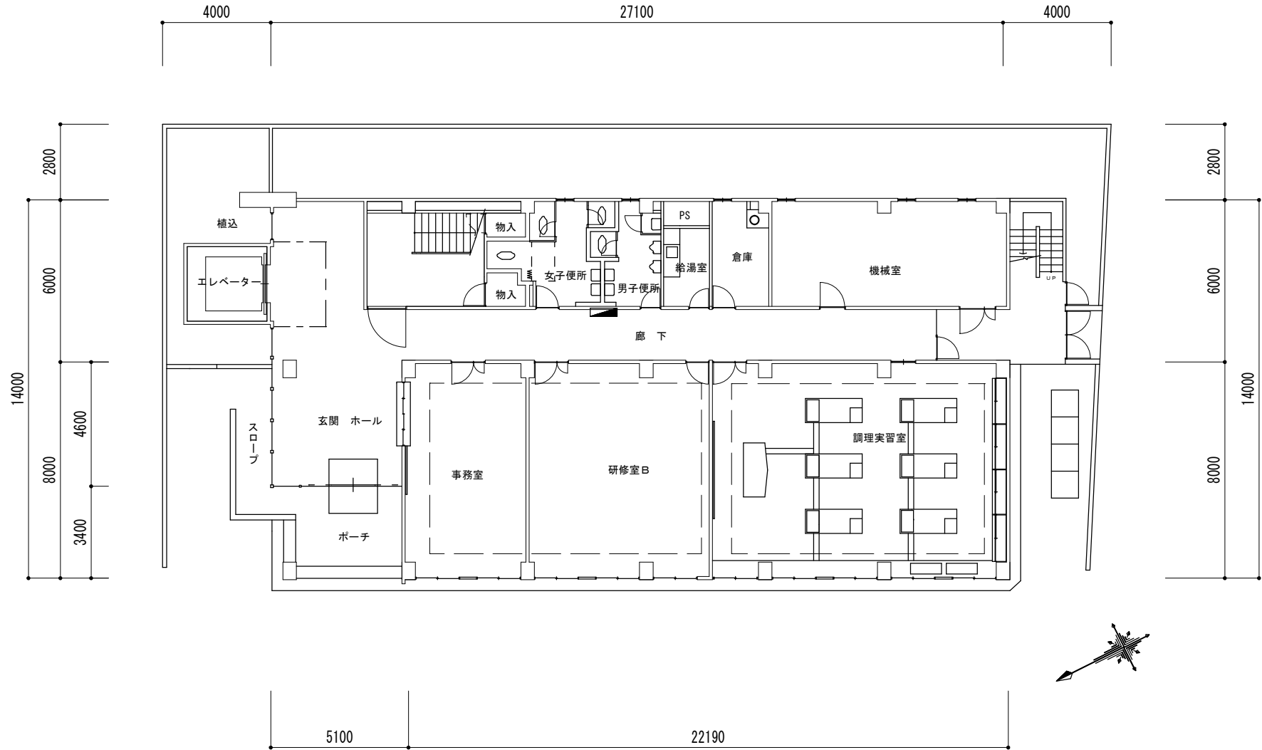
1階平面図
